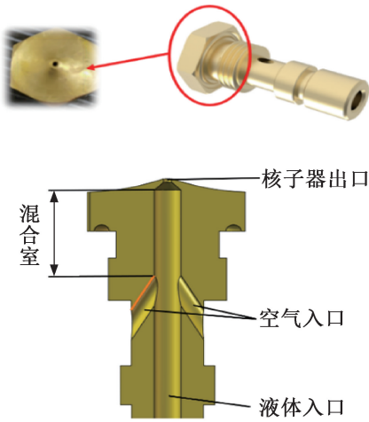
图5 核子器实物和内部结构
