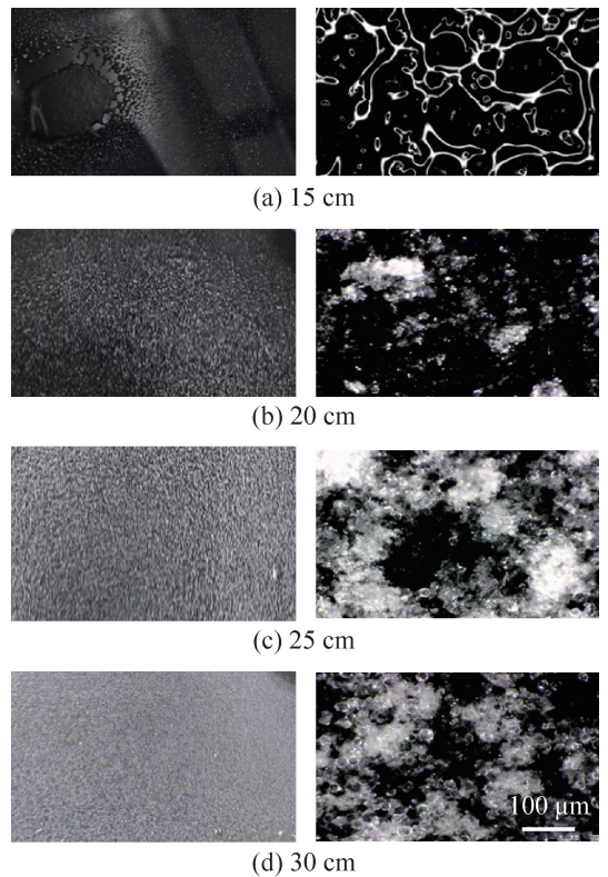
图7 不同落雪高度下雪晶宏观图和微观图
