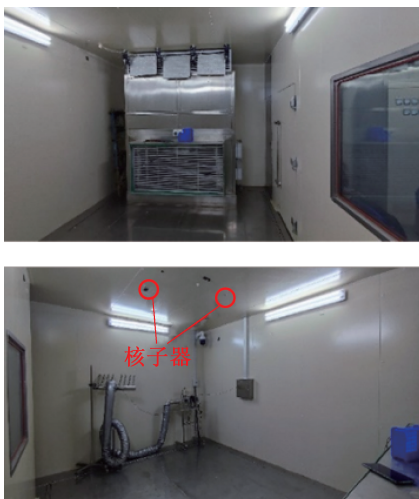
图 4 环境模拟室内景
