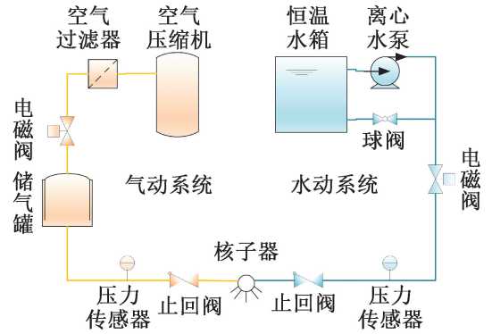
图 3 人工降雪实验系统
