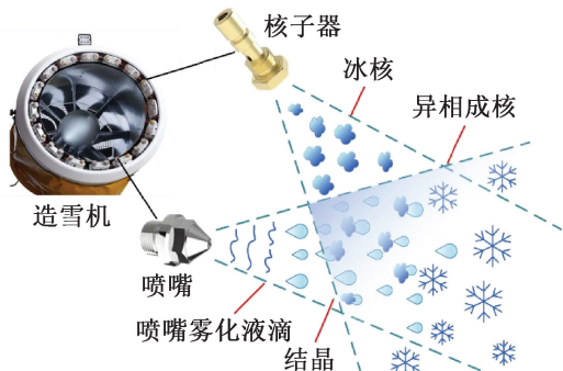
图1 人造雪的形成 Fig.1 Formation of artificial snow
