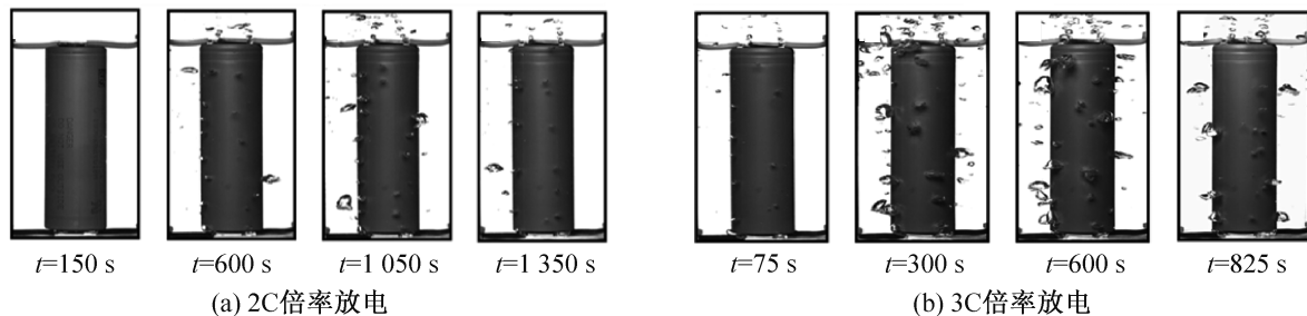
图 9 气液相变过程 [105]
