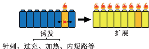
(c) 单体电池热失控引发相邻单体的热失控 [14]
