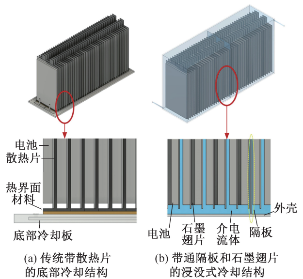
图 7 带翅片的浸没式结构 [91]
