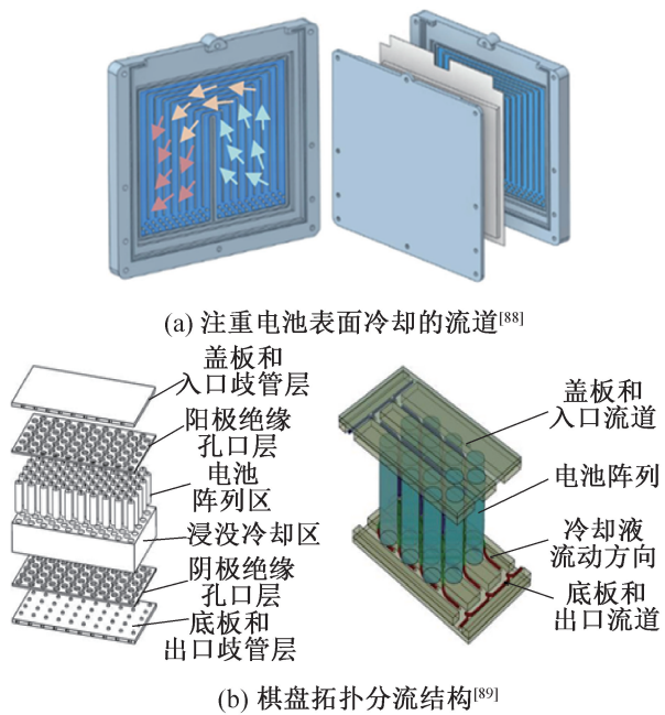
图 6 流道设计
