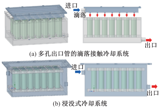
图 5 优化的浸没式冷却系统 [87]
