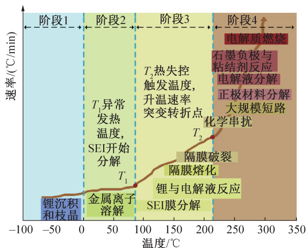
(a) 锂离子电池热失控机理及流程 [12]
