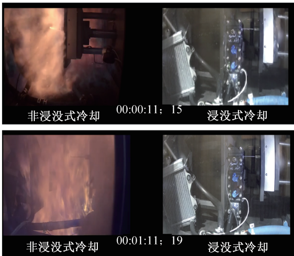
图 3 浸没液冷与非浸没液冷电池组穿刺实验对比 [48]
