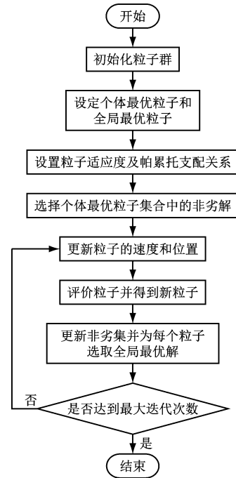
图 1 MOPSO 算法流程
