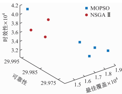
图4 帕累托解集
