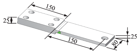
图5 焊接试验件尺寸(单位:mm)
