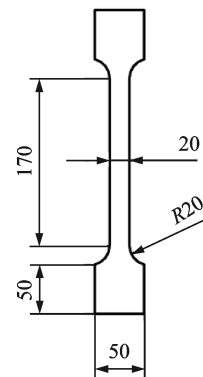
图1 拉伸试样的几何尺寸(单位:mm)
