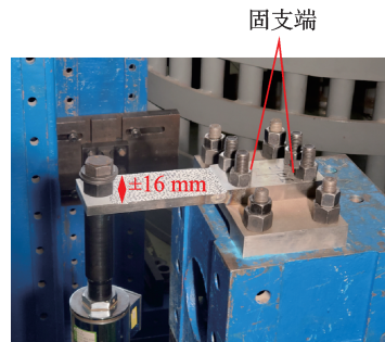
图6 焊接件安装情况
