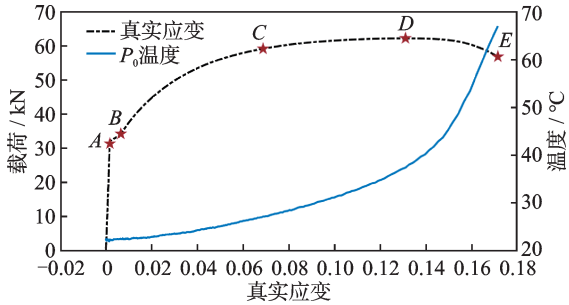
图3 拉伸试验中载荷与温度随真实应变的变化关系
