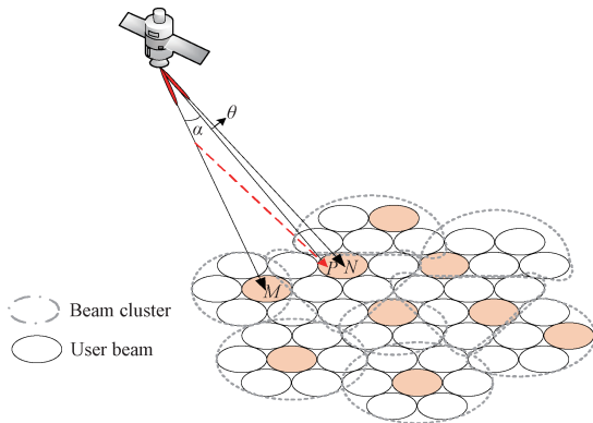
图 4 跳波束卫星通信系统干扰模型
