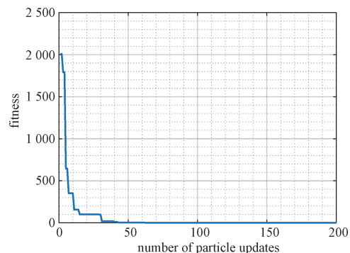
图 19 粒子群算法目标函数收敛曲线
