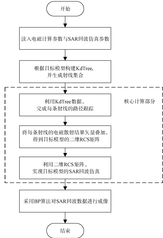
图1 传统的SAR回波仿真全流程
