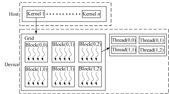
图 2 CUDA 线程层次结构
