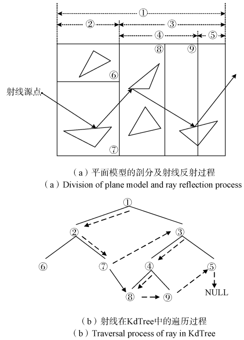
图4 平面模型中的射线追踪路径
