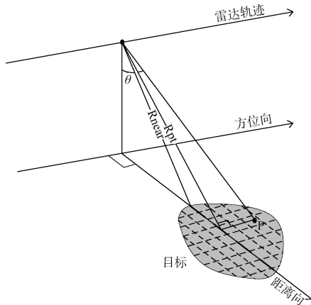
图 7 SAR 时域回波仿真几何图
