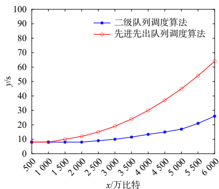
图 12 转发时延对比图
