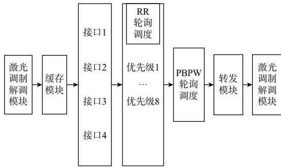
图3 数据帧经二级队列调度过程图
