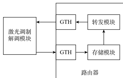
图 2 星上信息处理架构
