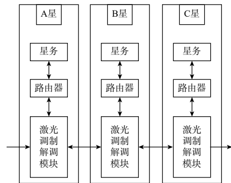
图1 星上数据处理过程图
