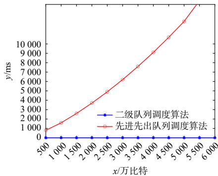
图 11 高优先级数据帧处理时间对比图
