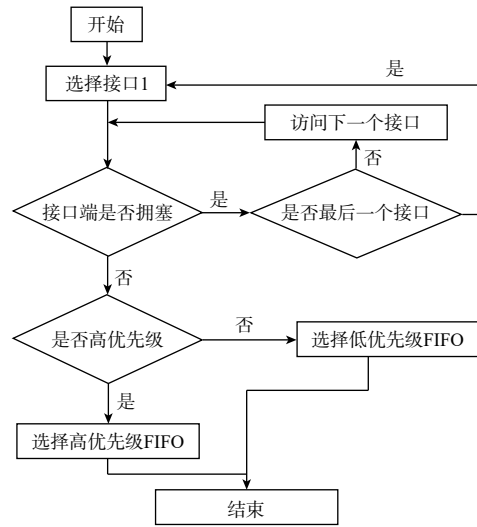
图4 RR轮询调度策略框图
