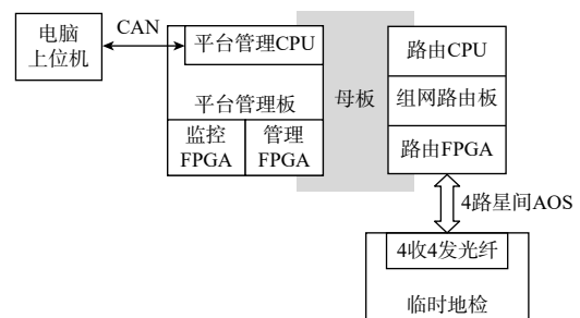
图 7 设备连接图
