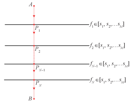
图3 M 个面的环境中的 N 阶射线
