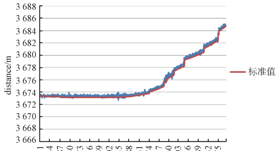
图 16 车速为 20 km/h 时距离对比曲线 Fig. 16 Distance contrast curve at 20 km/h
