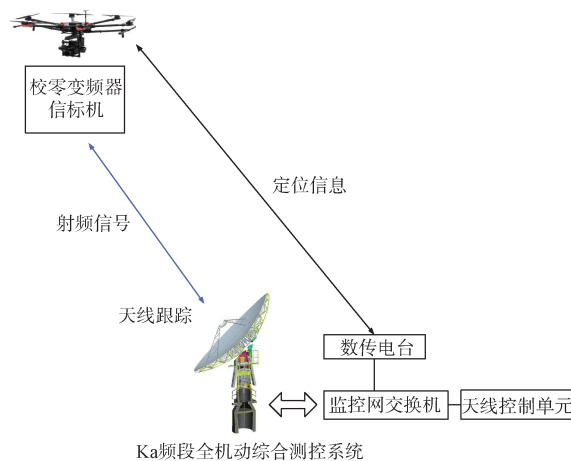
图 1 无人机标校原理图
