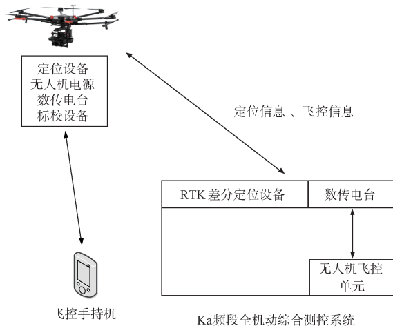
图2 无人机标校系统组成及布局
