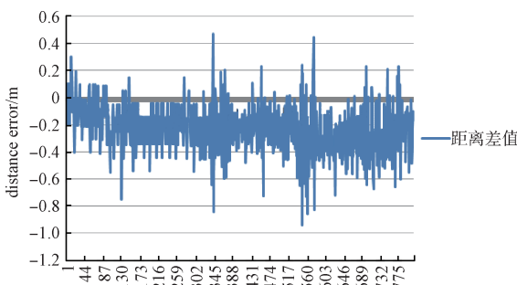
图 17 车速为 20 km/h 时距离误差曲线 Fig. 17 Distance error curve at 20 km/h
