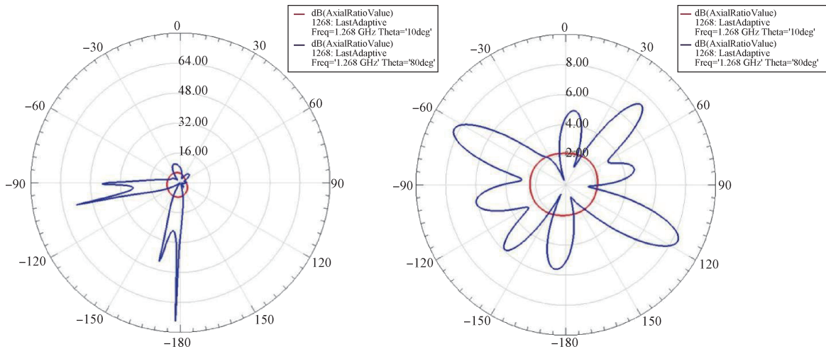
图 2 阵元 1 与阵元 2 的 HFSS 模型轴比
