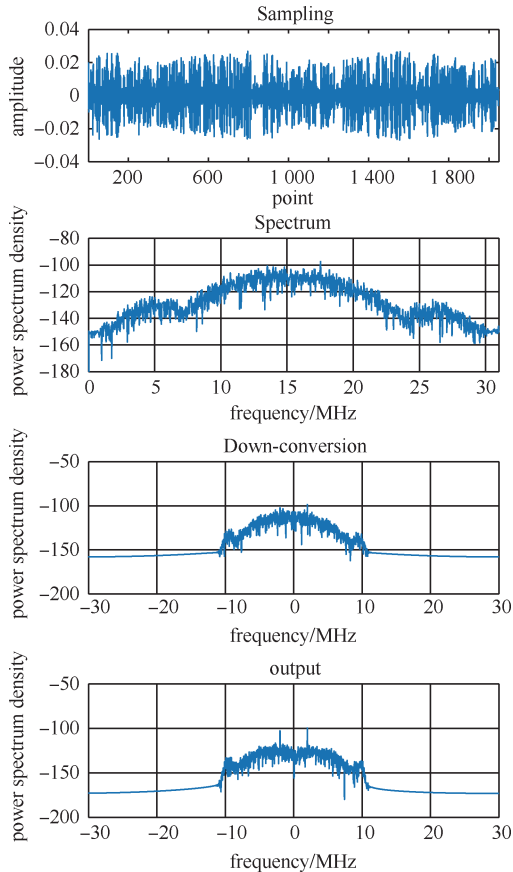
图9 实测4阵元阵列功率谱
