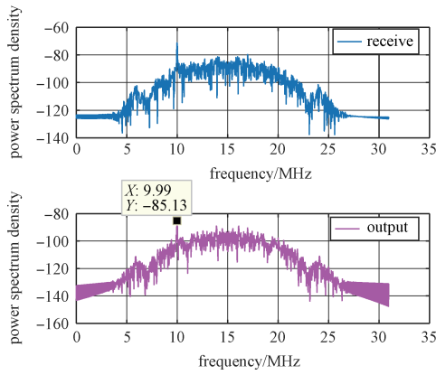
图 5 普通阵列输出信号功率谱
