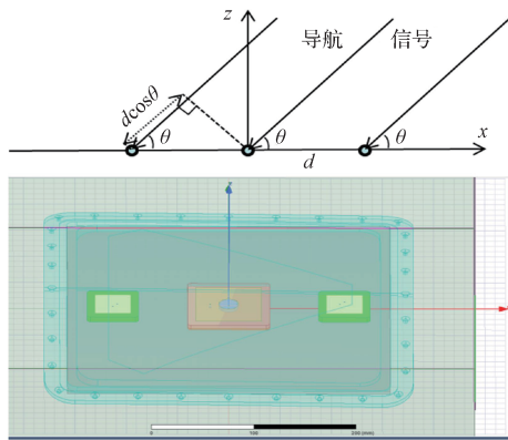
图 1 天线阵列 HFSS 模型
