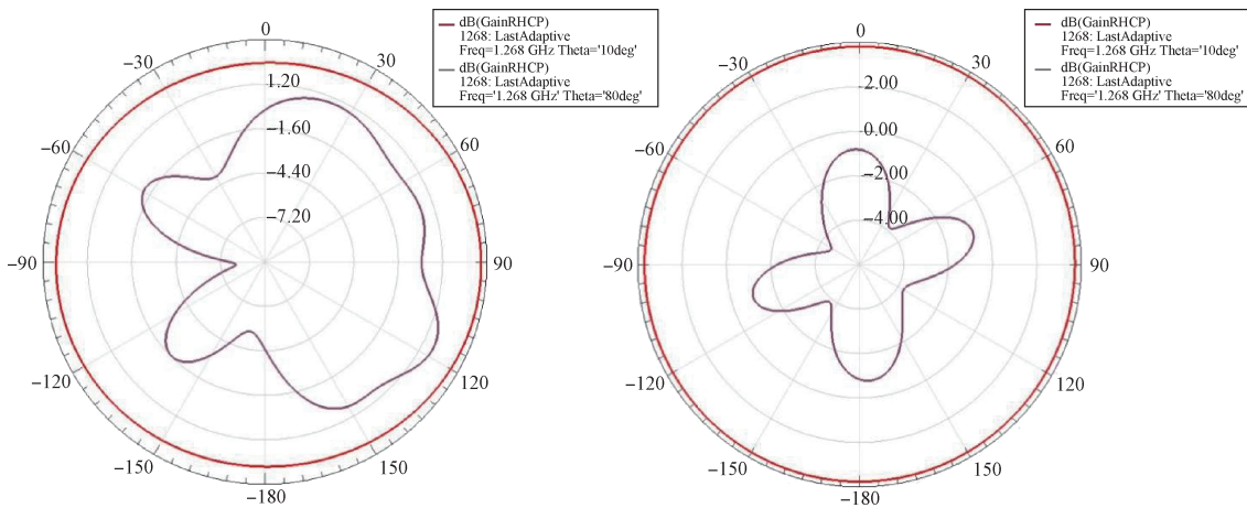
图3 阵元1与阵元2的HFSS模型接收增益
