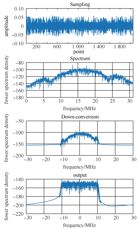
图10 实测4阵元双极化阵列功率谱
