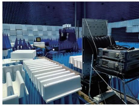
图 8 暗室测试环境
