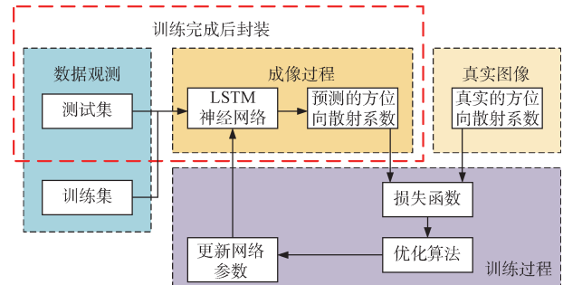
图3 基于LSTM神经网络的前视成像算法流程图
