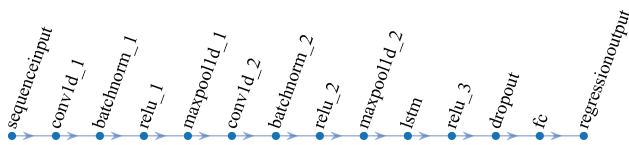
图2 CNN-LSTM神经网络结构
