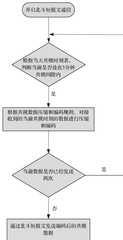
图 2 共视数据压缩传输流程图 Fig.2 Schematic diagram of common-view file
