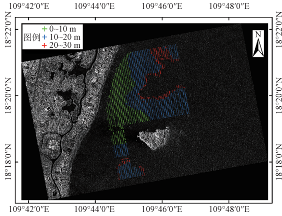
图6 反演水深
