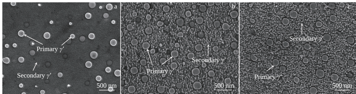
图3 GH4698合金热处理过程中晶内组织变化
