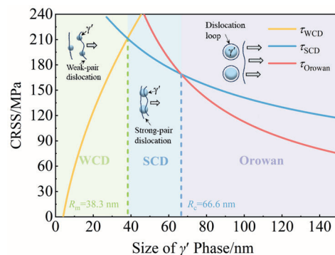
图13 临界分切应力随 \gamma' 相尺寸变化的理论值以及不同作用机制示意图
