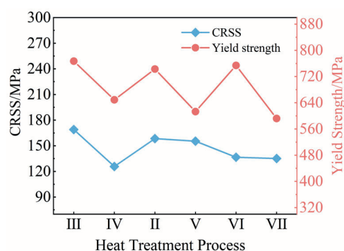
图14 各制度CRSS的理论值与实际测量屈服强度的比较
