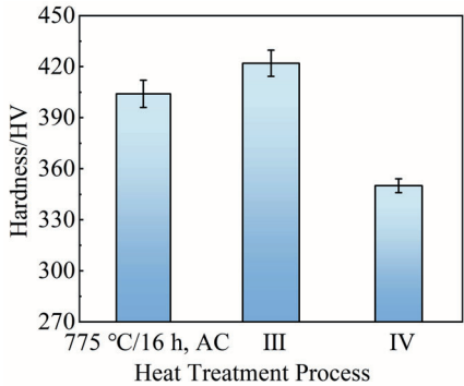
图8 GH4698 合金在不同热处理制度下的硬度
