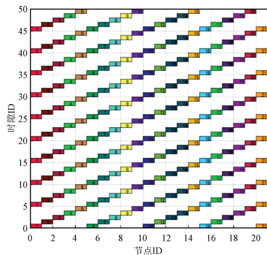
图 13 资源复用 TDMA 分配方式下节点占用时隙情况
