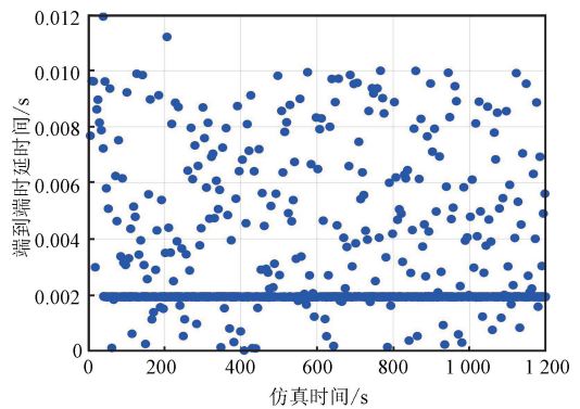
图 15 源节点 host[50] 队列等待时间 Fig. 15 Source node host[50] queue wait time
