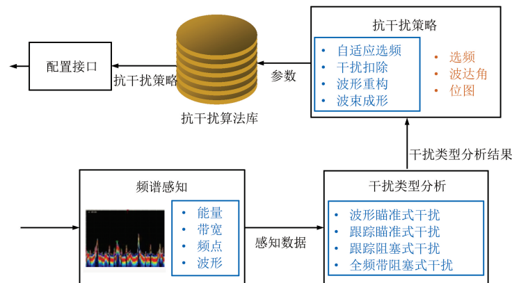
图5 基于频谱感知的综合抗干扰机制示意
