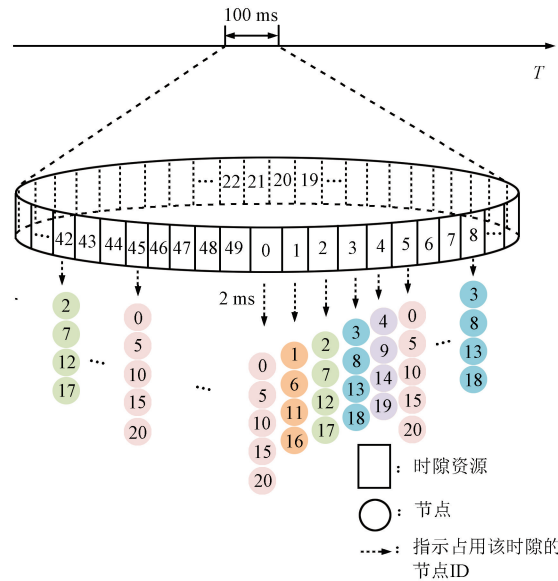
图 12 考虑资源复用的 TDMA 方案
