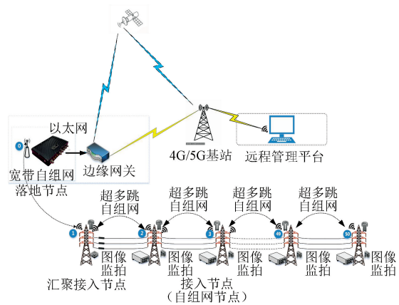
图 19 超多跳自组网在线监控系统框图 Fig. 19 Online monitoring system of the ultra-multi-hop ad hoc network
