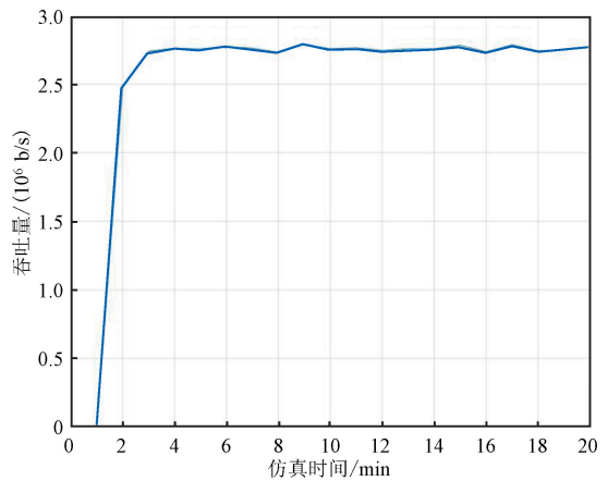
图 16 50 跳网络吞吐量 Fig. 16 50-hop network throughput
