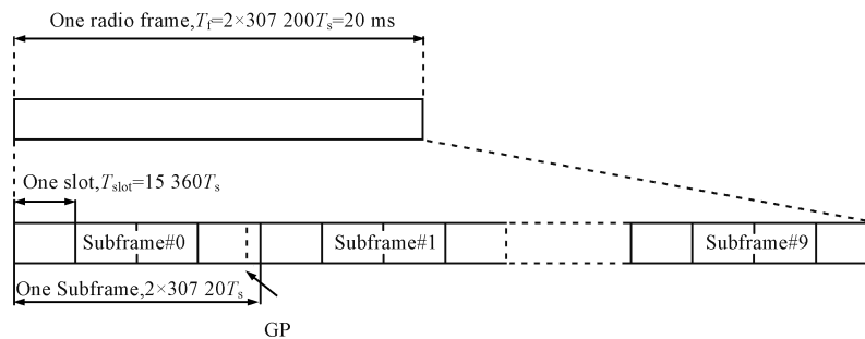
图 1 帧结构
