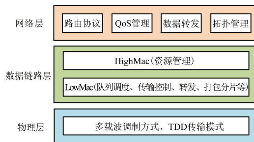
图8 宽带自组织波形架构
