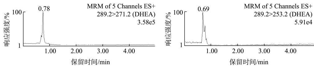
图 4 实际样品的液相色谱-质谱谱图
