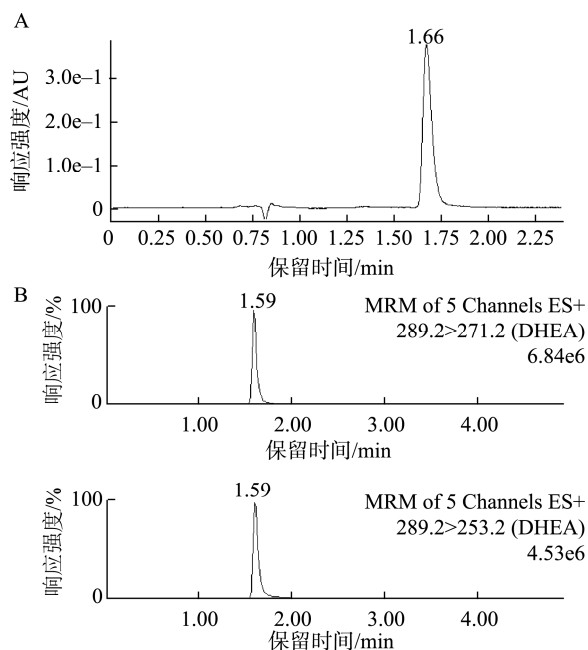
注: A. LC-二极管阵列检测色谱图(50 µg/mL); B. LC-MS 谱图(1 ng/mL)(上下两图分别是 DHEA 的定量离子对和定性离子对)。
