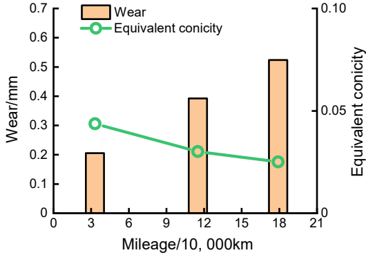
Wuhan-Guangzhou HSR (b)
