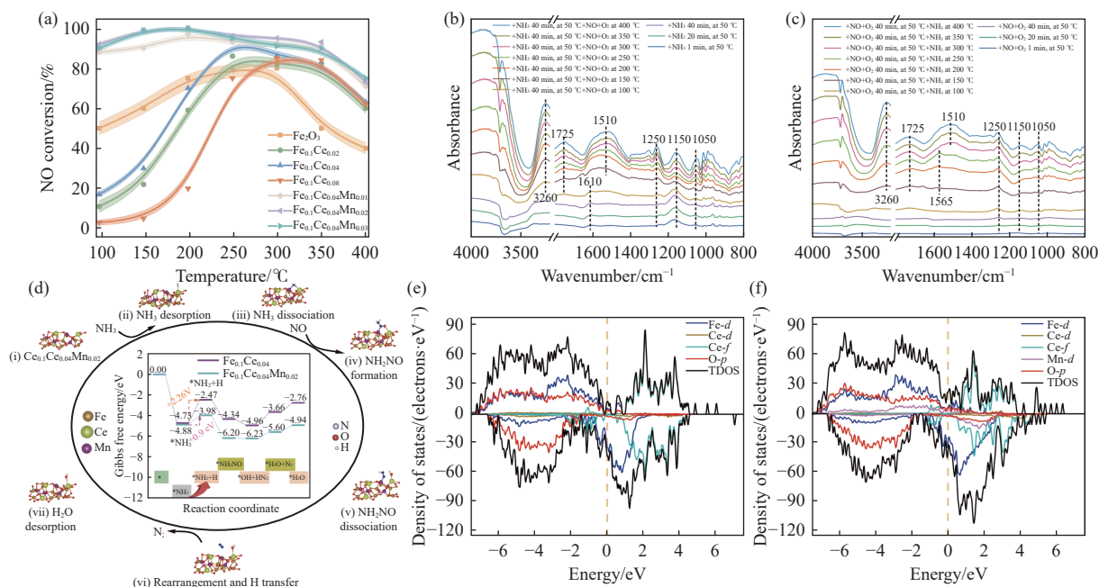
图 2 Fe-Ce-Mn 催化剂 \text{NH}_3 -SCR 性能与机理解析: (a) \text{Fe}_2\text{O}_3 、 \text{Fe}_{0.1}\text{Ce}_x 与 \text{Fe}_{0.1}\text{Ce}_{0.04}\text{Mn}_y 催化剂 NO 转化率随温度变化; (b) \text{Fe}_{0.1}\text{Ce}_{0.04}\text{Mn}_{0.02} 在预吸附 \text{NH}_3 后通入 \text{NO} + \text{O}_2 的原位 DRIFTS 光谱谱图; (c) \text{Fe}_{0.1}\text{Ce}_{0.04}\text{Mn}_{0.02} 在预吸附 \text{NO} + \text{O}_2 后通入 \text{NH}_3 的原位 DRIFTS 光谱谱图; (d) \text{Fe}_{0.1}\text{Ce}_{0.04} 与 \text{Fe}_{0.1}\text{Ce}_{0.04}\text{Mn}_{0.02} 上 \text{NH}_3 -SCR 反应路径及吉布斯自由能变化; (e) \text{Fe}_{0.1}\text{Ce}_{0.04} 的投影态密度(PDOS); (f) \text{Fe}_{0.1}\text{Ce}_{0.04}\text{Mn}_{0.02} 的投影态密度(PDOS)
