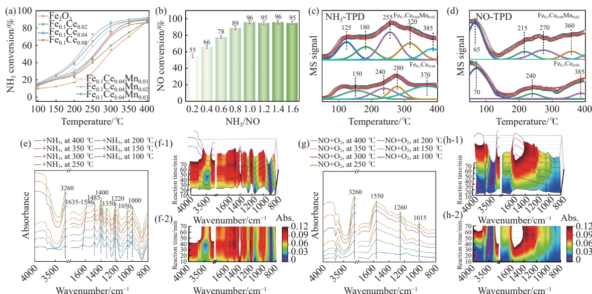
图3 Fe-Ce-Mn 基催化剂 \text{NH}_3 -SCR 活性及表面吸附行为: (a) 不同催化剂 \text{NH}_3 转化率随温度变化; (b) 200 °C 时 \text{NH}_3/\text{NO} 摩尔比对 \text{Fe}_{0.1}\text{Ce}_{0.04}\text{Mn}_{0.02} 催化剂 NO 转化率的影响; (c) \text{Fe}_{0.1}\text{Ce}_{0.04} 与 \text{Fe}_{0.1}\text{Ce}_{0.04}\text{Mn}_{0.02} 的 \text{NH}_3 -TPD 谱图; (d) \text{Fe}_{0.1}\text{Ce}_{0.04} 与 \text{Fe}_{0.1}\text{Ce}_{0.04}\text{Mn}_{0.02} 的 NO-TPD 谱图; (e) \text{Fe}_{0.1}\text{Ce}_{0.04}\text{Mn}_{0.02} 在预吸附 \text{NH}_3 后通入 \text{NO} + \text{O}_2 的原位 DRIFTS 光谱谱图; (f-1, f-2) 对应(e) 的三维及等高线 DRIFTS 谱图; (g) \text{Fe}_{0.1}\text{Ce}_{0.04}\text{Mn}_{0.02} 在预吸附 \text{NO} + \text{O}_2 后通入 \text{NH}_3 的原位 DRIFTS 谱图; (h-1, h-2) 对应(g) 的三维及等高线 DRIFTS 谱图
