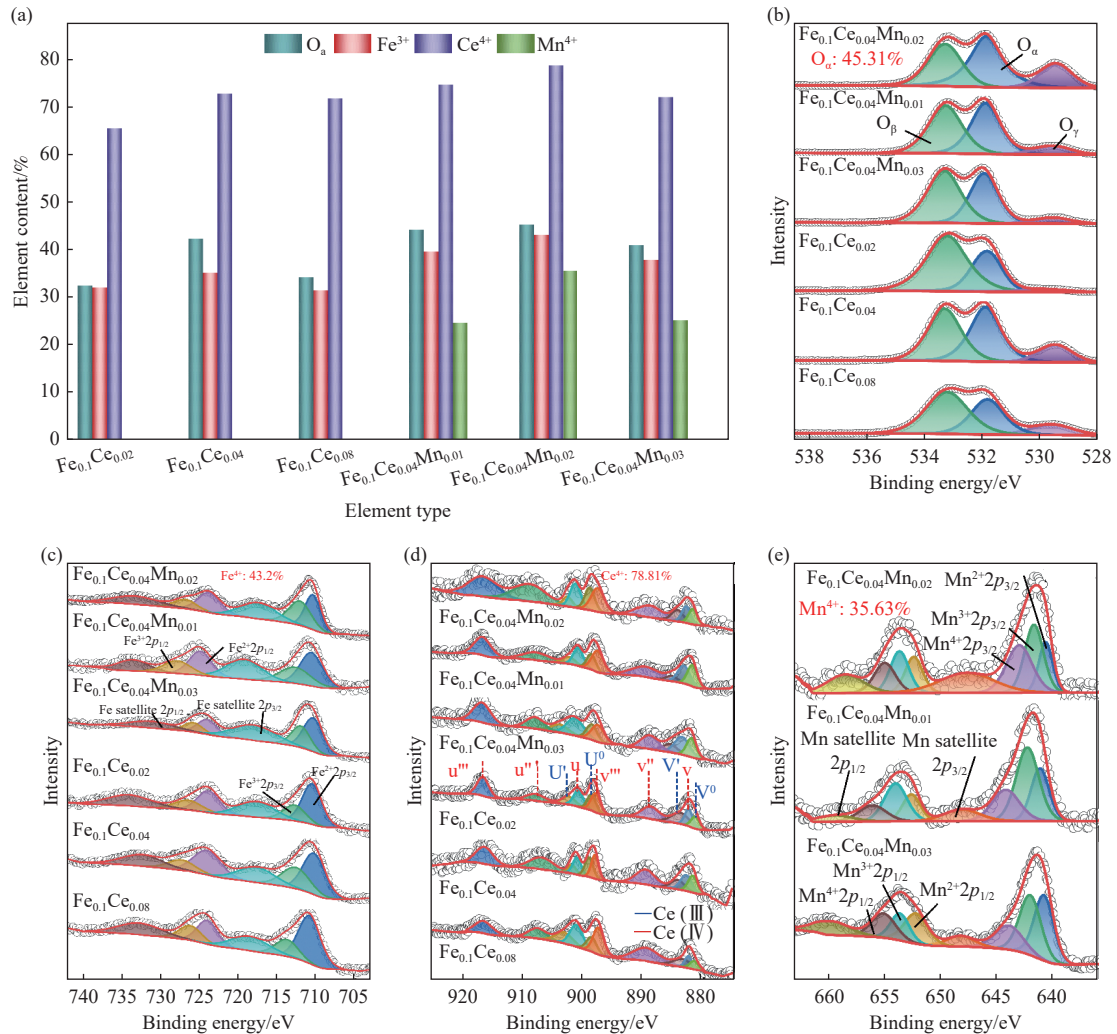
图 5 (a) XPS 光谱汇总; (b) O 1s 光谱; (c) Fe 2p 光谱; (d) Ce 3d 光谱; (e) Mn 2p 光谱 Fig. 5 (a) Summary of the XPS spectra; XPS spectra of (b) O 1s; (c) Fe 2p; (d) Ce 3d and (e) Mn 2p
