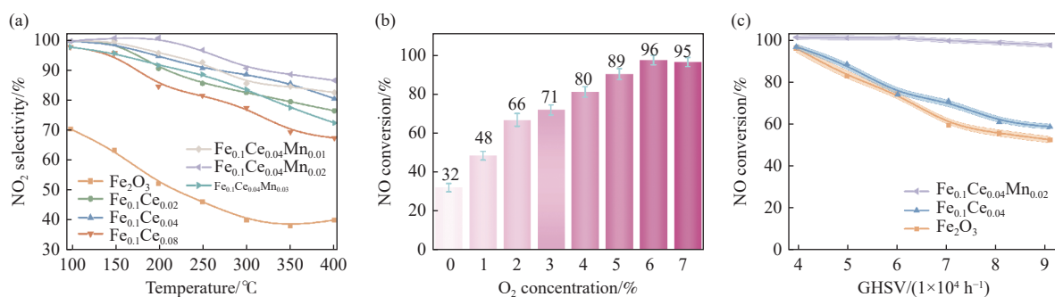
图 4 Fe-Ce-Mn 催化剂 \text{NH}_3 -SCR 选择性及反应条件影响: (a) 不同催化剂 \text{N}_2 选择性随温度变化; (b) 200 °C 时 \text{O}_2 体积分数对 NO 转化率的影响; (c) 200 °C 时空速对 NO 转化率的影响
