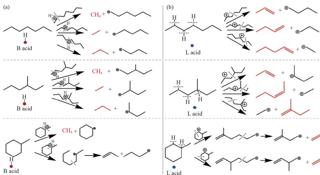
图 5 不同结构 C 7 烃在改性 ZSM-5 的 B 酸和 L 酸上的单分子裂解反应机理示意图
