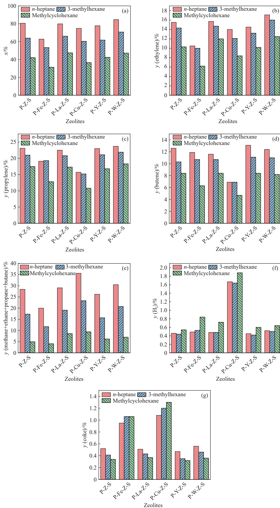
图 3 改性 ZSM-5 分子筛催化不同结构 C_7 烃裂解反应的转化率及主要产品收率
