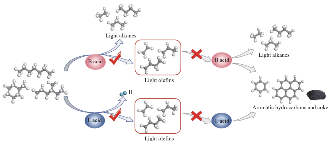
图 6 不同结构 C 7 烃在改性 ZSM-5 上的催化裂解反应路径示意图
