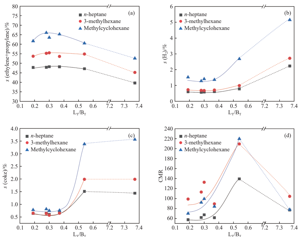
图 4 不同结构 C 7 烃催化裂解主要产物选择性及 CMR 随 L_T/B_T 的变化
