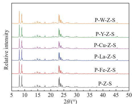
图 1 水热处理后改性 ZSM-5 分子筛的 XRD 谱图 Fig. 1 XRD patterns of modified ZSM-5 molecular sieves by hydrothermal treatment
