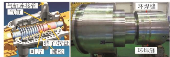
a) 螺栓连接转子 b) LTES700R焊接转子
