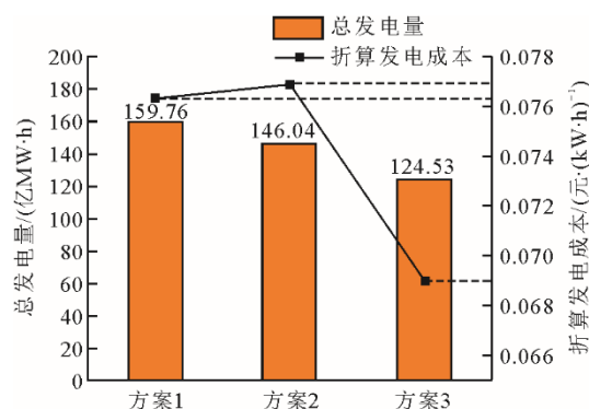
图3 不同改造方案下总发电量和发电成本预测
