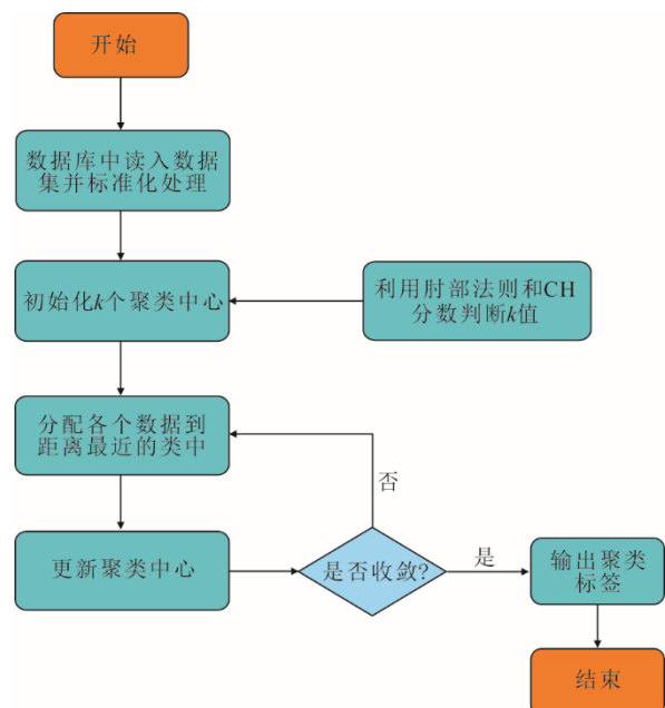
图1 K-means 聚类算法流程
