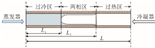
图2 移动边界模型示意
