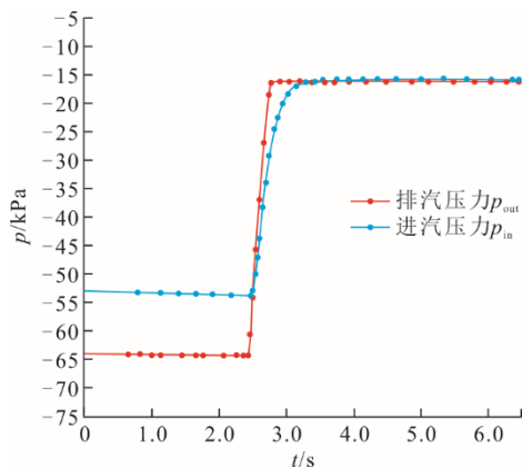
图3 现场汽轮机紧急停机进排汽压力变化曲线
