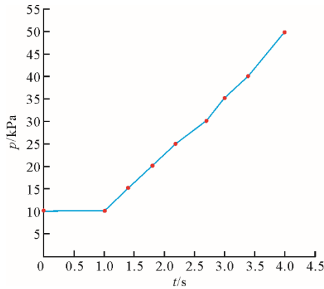
图2 汽轮机排汽压力-时间曲线
