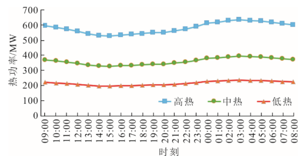
a) 热负荷
