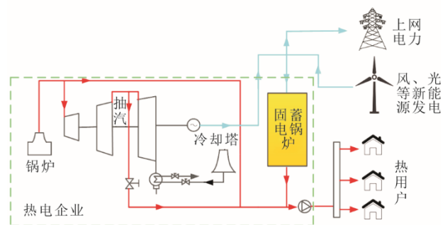
图 2 固蓄电锅炉电-热传输情况
