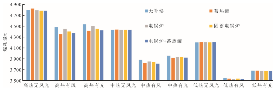
图 9 机组配置不同供热补偿设备日内煤耗量统计
