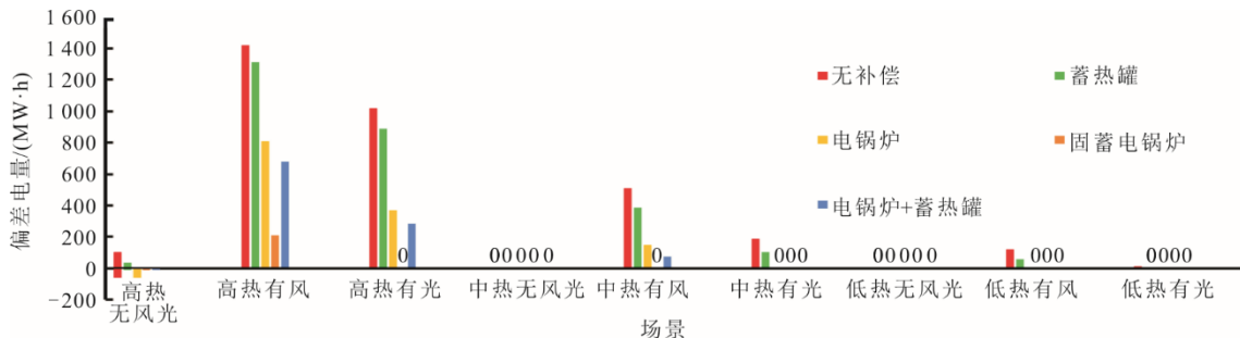
图 7 机组配置不同供热补偿设备日内偏差电量统计
