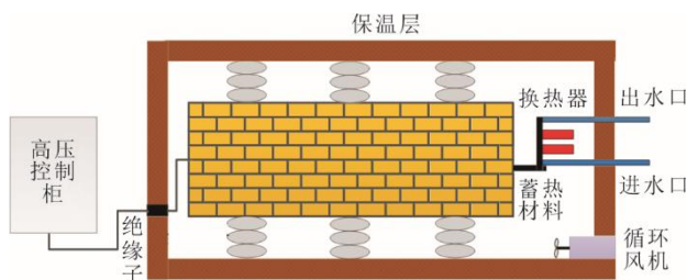
图 1 固蓄电锅炉原理
