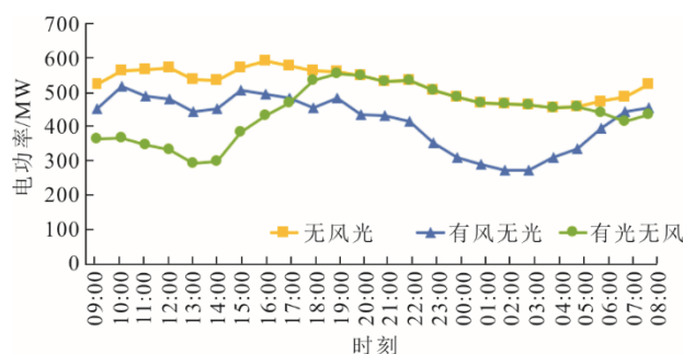
b) 电负荷
