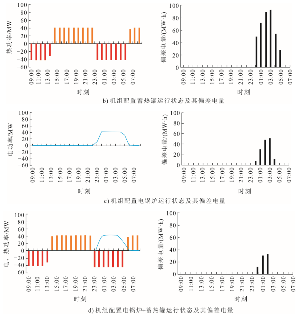
图 8 供热补偿设备的运行状态与偏差电量
