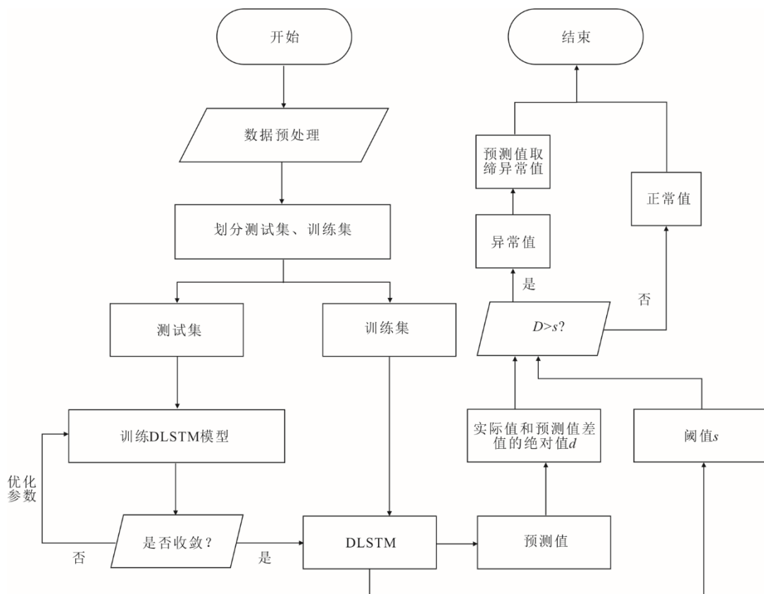
图 3 DLSTM 数据清洗模型流程
