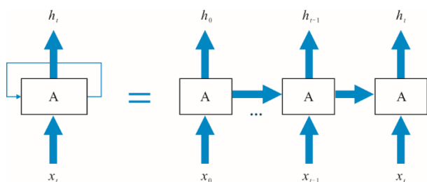
图 1 RNN 展开结构
