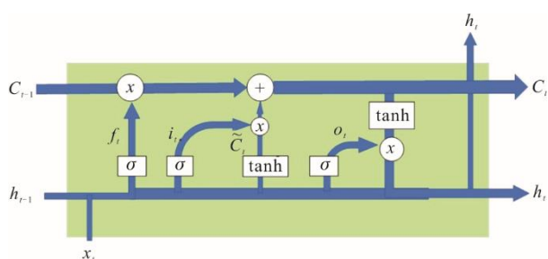
图 2 LSTM
