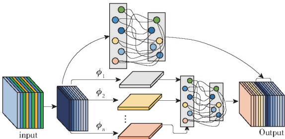
图 4 LNN GhostDynamicConv (LGC) 模块 Fig. 4 LNN GhostDynamicConv (LGC) module
