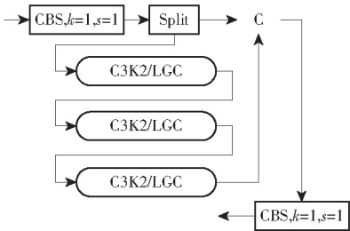
图 3 C3K2 - LGC 模块 Fig. 3 C3K2 - LGC module
