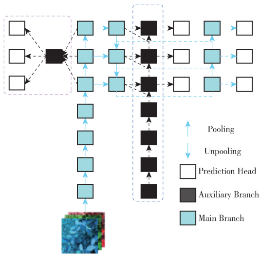
图 6 PGI 结构图
