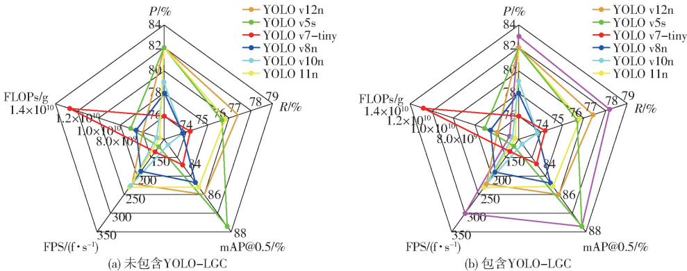
图 9 不同模型雷达图 Fig. 9 Radar charts of different models
