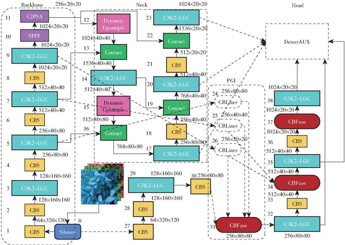
图2 YOLO-LGC 模型
