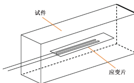
图 3 试件预埋应变片示意图
