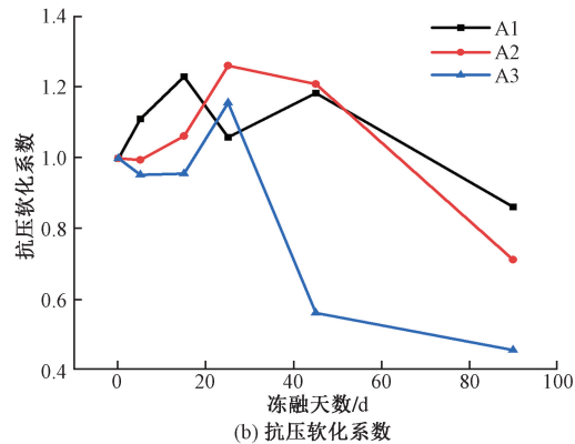
(b) 抗压软化系数
