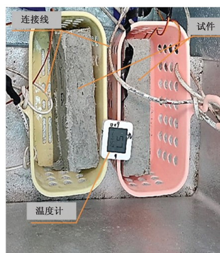
图 2 冻融试件测试示意图
