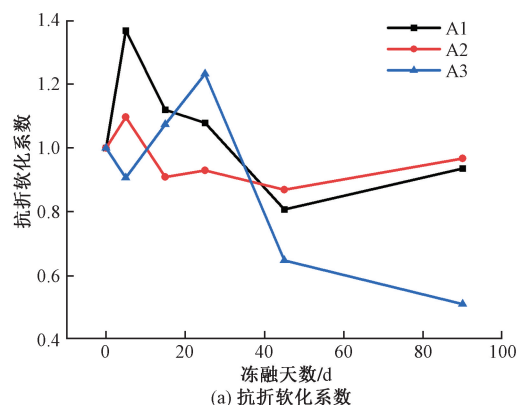
(a) 抗折软化系数
