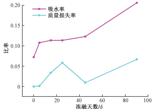
图 12 碱性环境质量损失率与吸水率
