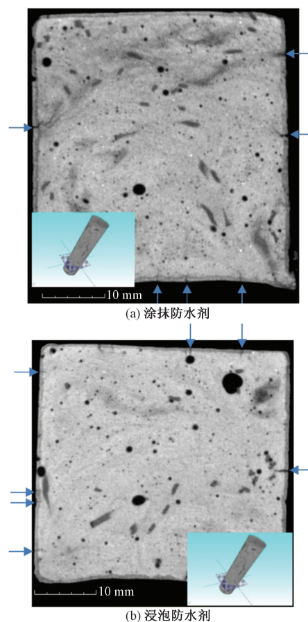
图 15 冻融 45 d 后 CT 扫描图
