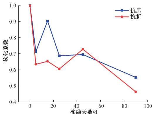
图 11 碱性环境软化系数
