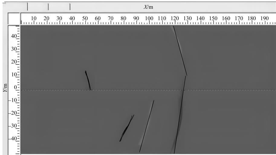
图2 煤矿 83207 内错尾巷纵波提取的反射层
