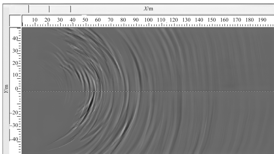
图 1 煤矿 83207 内错尾巷纵波深度偏移剖面
