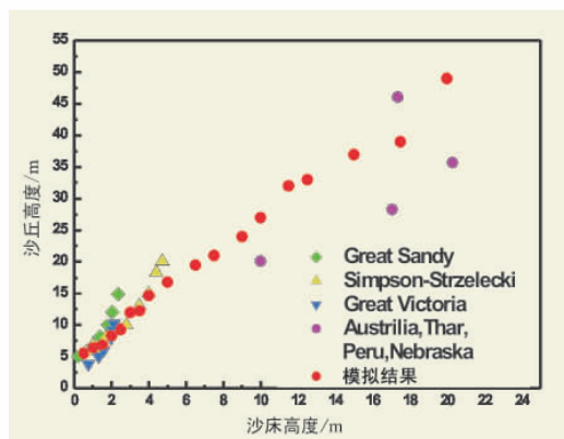
图 4 沙丘高度随沙床高度的变化
