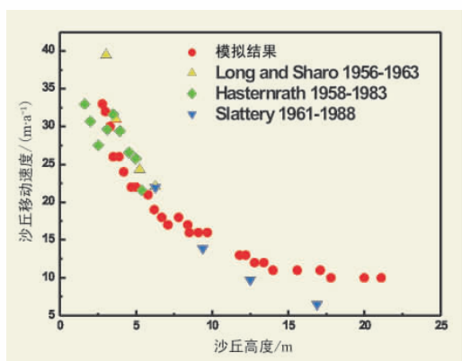
图 3 沙丘移动速度随高度的变化
