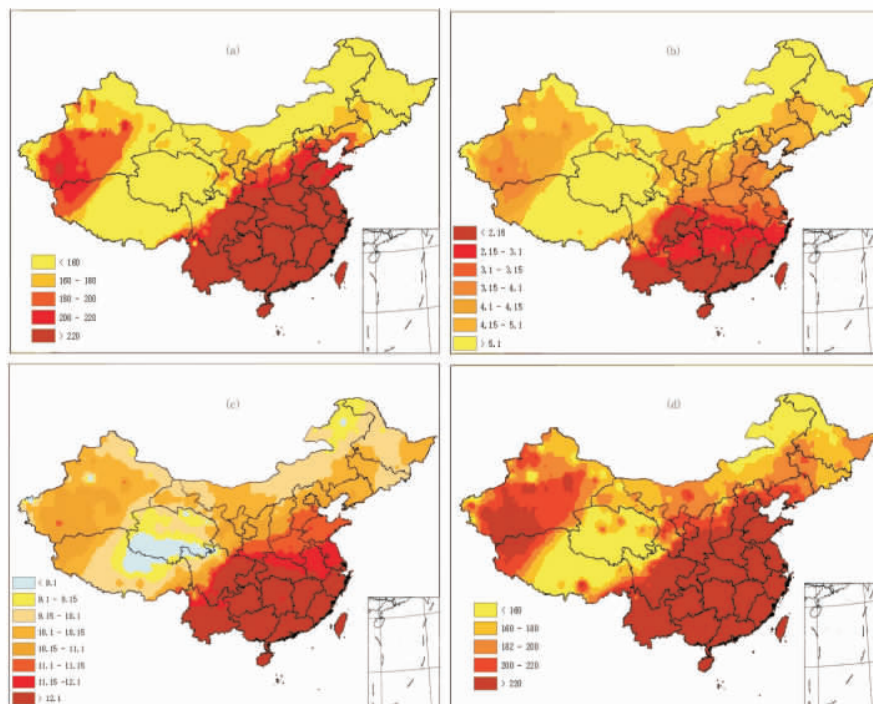
(a) 近 45 a 我国无霜期平均值分布图; (b) 近 45 a 我国终霜日平均值分布图;
