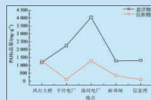
悬浮物和沉积物中 \Sigma PAHs 沿程分布
