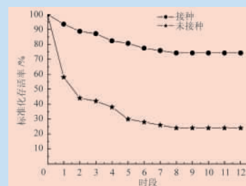
猪血木幼苗存活率曲线
