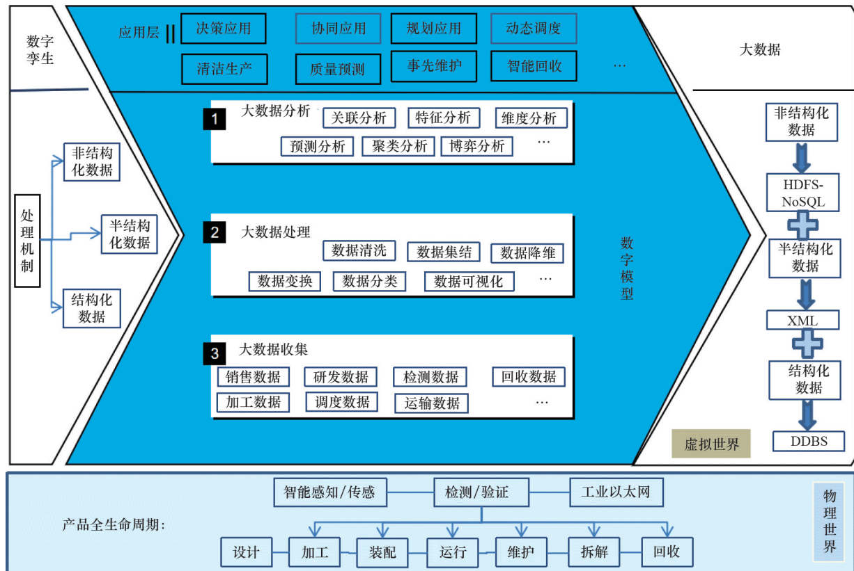
图2 数字孪生驱动的大数据制造服务模式体系架构
