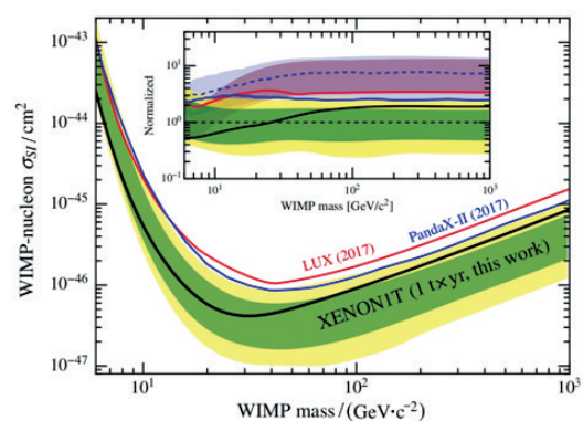
图5 液氙实验对自旋无关的暗物质和核子相互作用的最新限制 [10]
