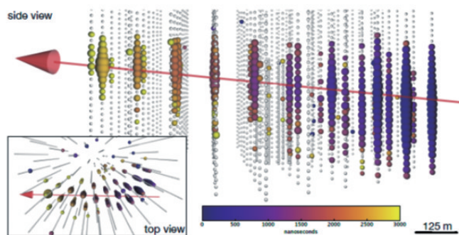
图3 冰立方实验观测的耀变体高能中微子信号(IceCube-170922A) [5]
