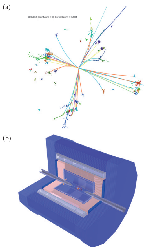
图11 CEPC上的典型希格斯粒子示例(a) 以及基线探测器(b)
