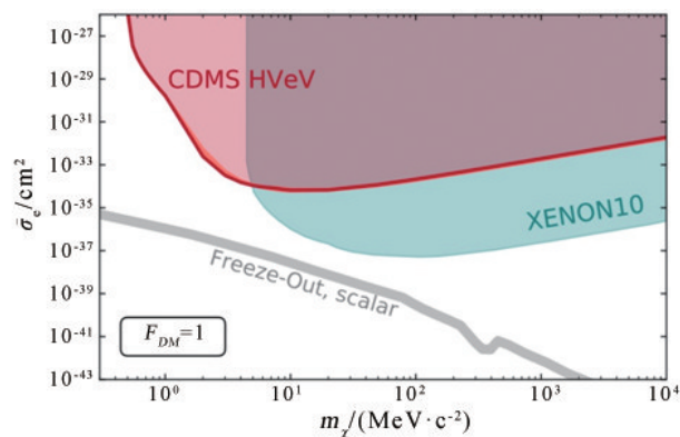
图7 CDMS HVeV实验对暗物质和电子相互作用的最新限制 [17]
