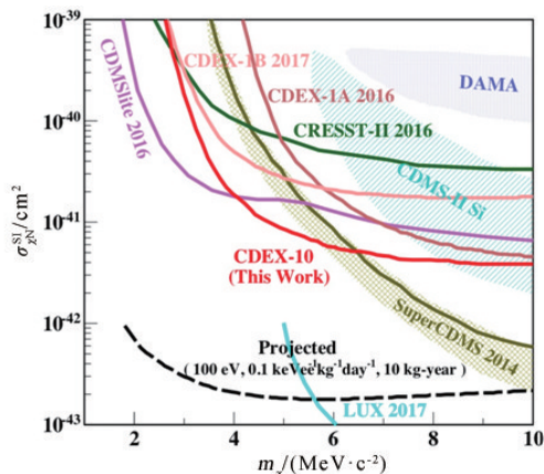
图6 中国CDEX实验对自旋无关小质量暗物质和核子相互作用的最新限制 [13]
