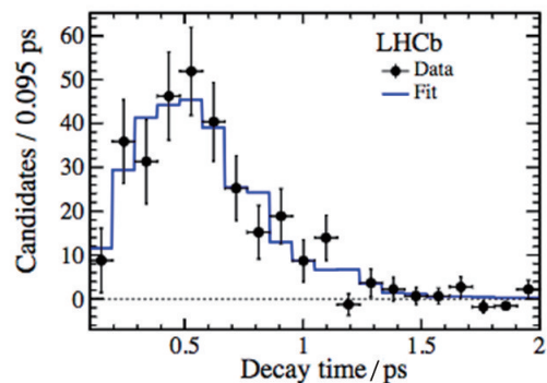
图9 \Xi_{cc}^{++} 寿命测量
