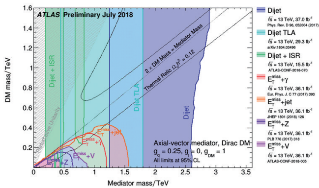
图8 ATLAS实验对暗物质和中间传播子参数空间的实验限制(图片来源:ATLAS实验组)
