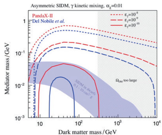
图4 中国 PandaX 实验对自相互作用暗物质模型的最新限制 [9]
