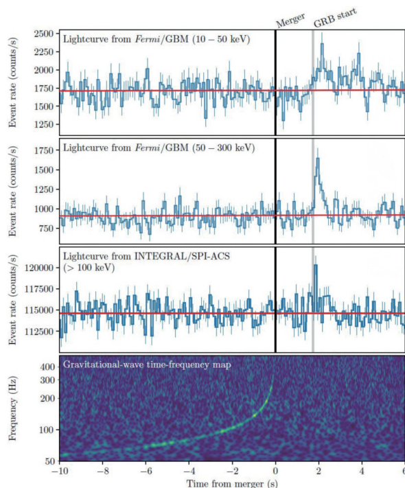
图 1 LIGO 引力波信号结束的时间和伽玛暴的开始时间相差大约 2 s (图片来源: LIGO-VIRGO)
