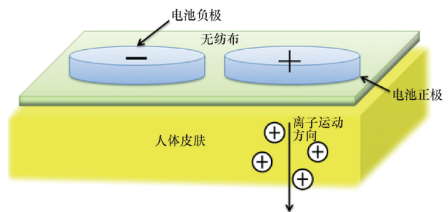
图4 离子电渗透示意
