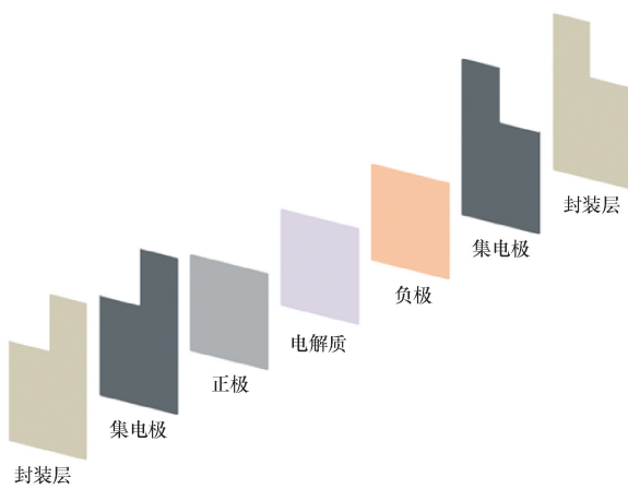
图1 薄膜纸电池组成结构
