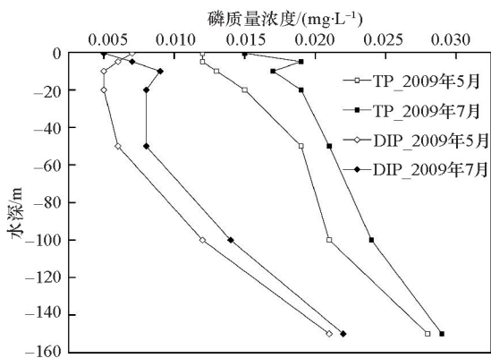
图4 水体中磷的垂直分布特征
