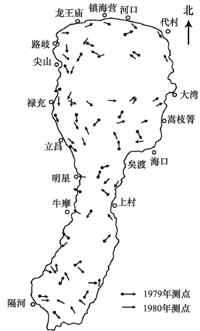
图3 抚仙湖实测流场图
