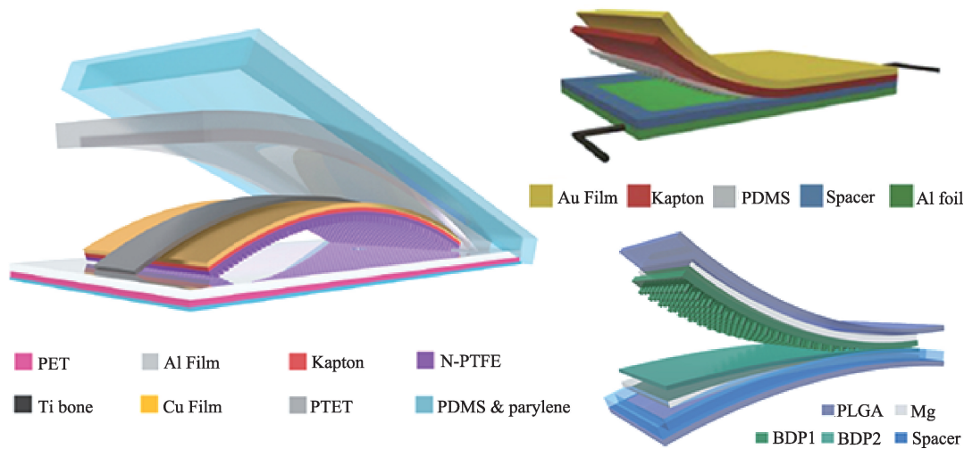
图 4 不同结构的 iTENG
