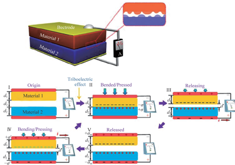
图7 iTENG 工作原理
