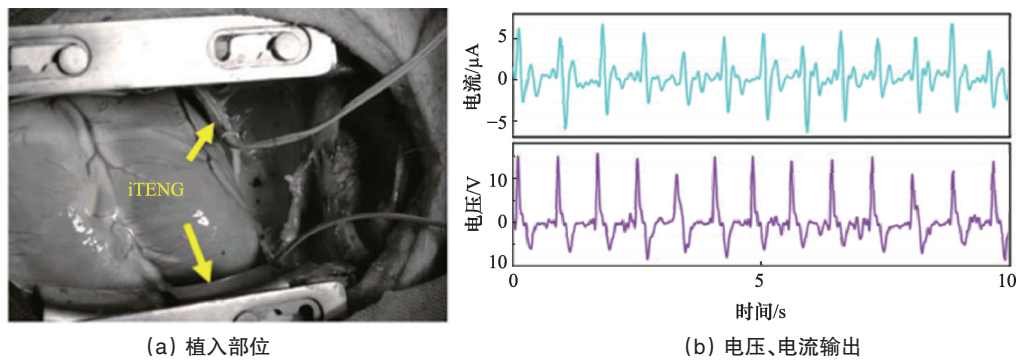
图9 植入到小鼠体内iTENG电信号输出图
