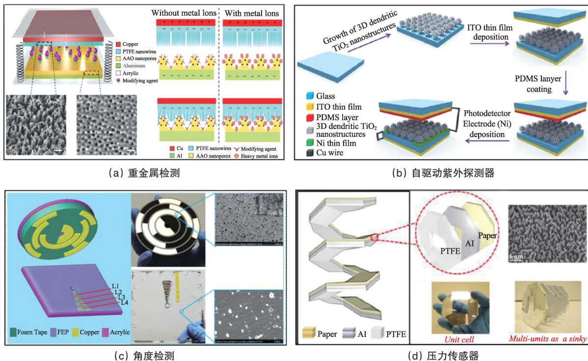
图3 TENG作为自驱动传感器的应用
