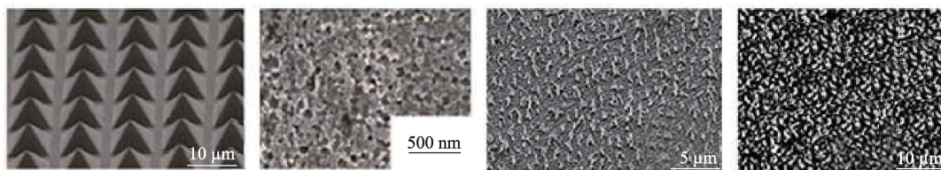
图 5 iTENG 不同材料摩擦层纳米结构扫描电子显微镜图
