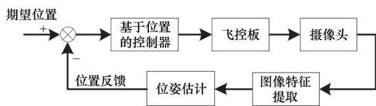
图 1 PBVS 的基本结构
