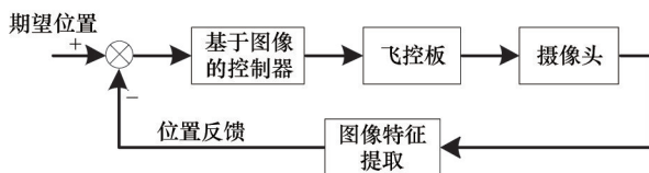
图 2 IBVS 的基本结构
