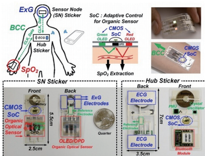
图3 血氧饱和度及生物电信号检测系统
