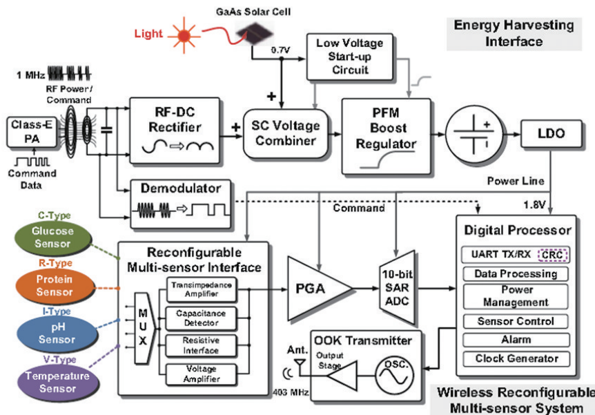
图1 无线可重构多传感器片上系统
