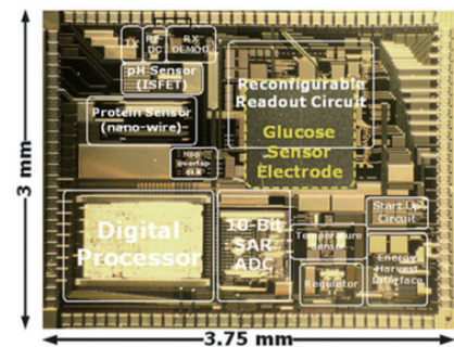
图2 可重构多传感器片上系统显微照片
