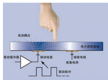
(b) 电容式触摸屏
