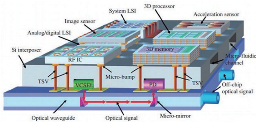
图 17 TSV 技术实现 CMOS、MEMS 以及光电子电路三维混合集成
