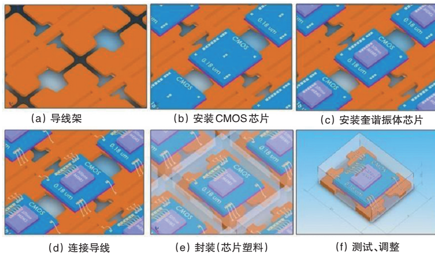
图 16 晶振封装技术
