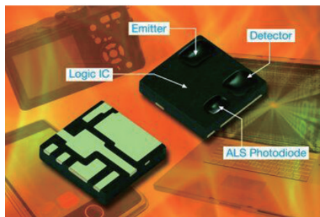
图10 接近和环境光传感器
