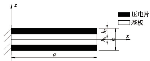
图4 双压电片悬臂梁结构
