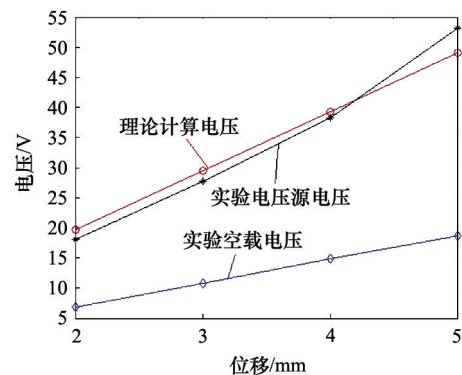
图6 3种电压比较曲线
