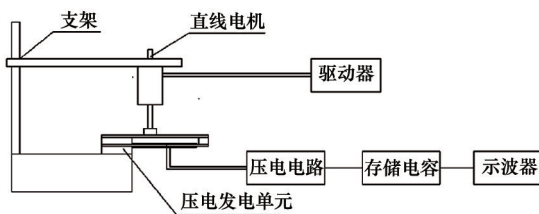
图5 振动实验装置示意
