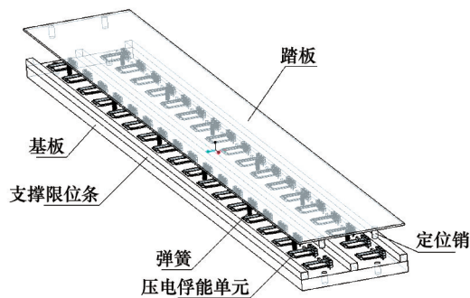
图1 压电发电装置整体结构
