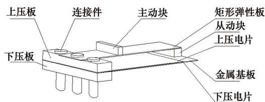
图2 压电发电单元
