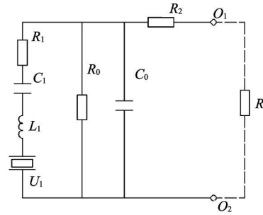
图3 压电片等效发电电路
