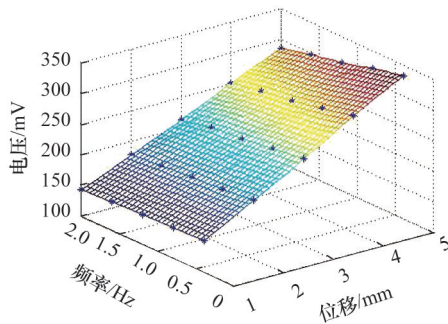
图7 电容电压与激励位移和频率关系
