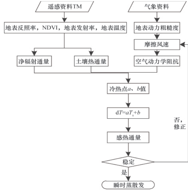
图 1 瞬时蒸散发估算流程图
