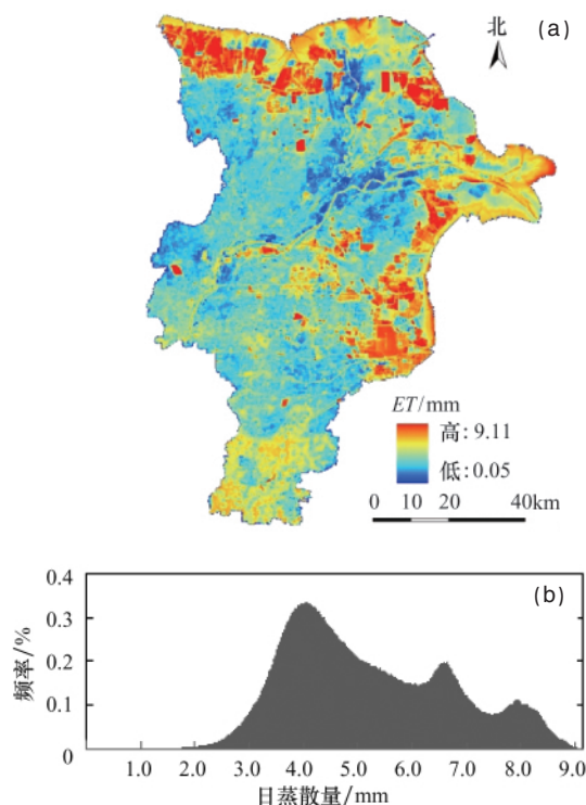
图2 2009年6月4日东营市日蒸散发量空间分布图(a)和频率分布图(b)
