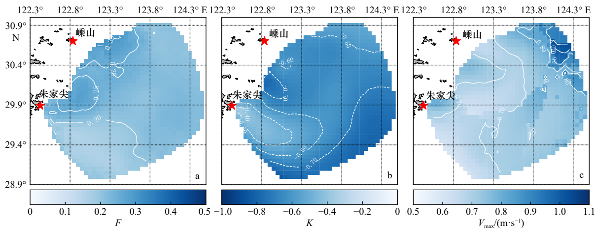
图 5 F 值 (a)、 K 值 (b) 和 V_{max} 值 (c) 分布
