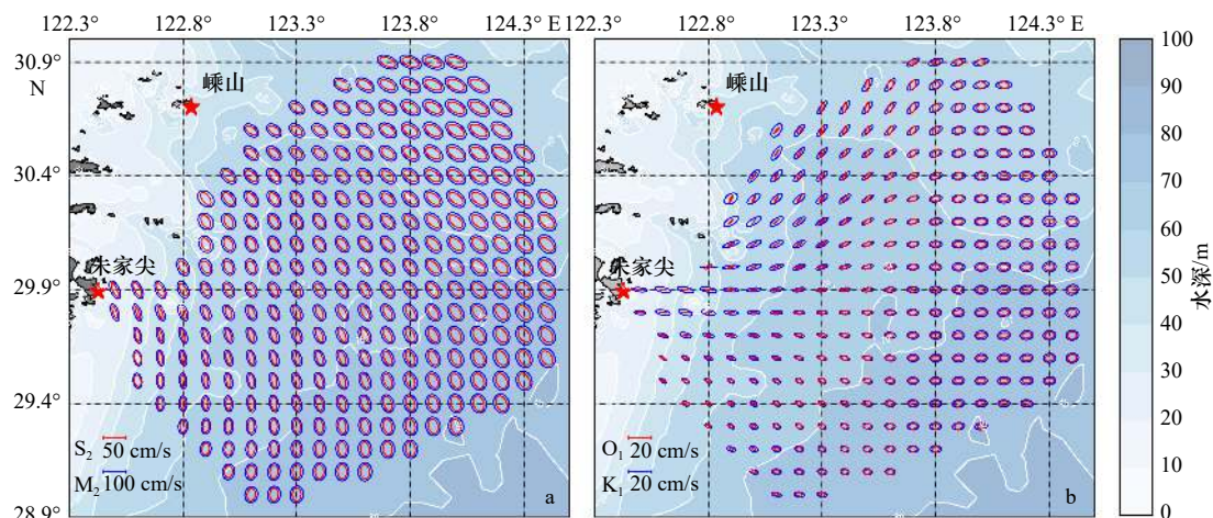
图 4 M_2 、 S_2 潮流椭圆 (a) 和 K_1 、 O_1 潮流椭圆 (b)
