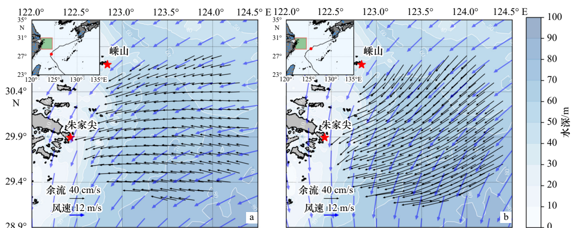
图 9 台风靠近与离开时刻余流场与风场
