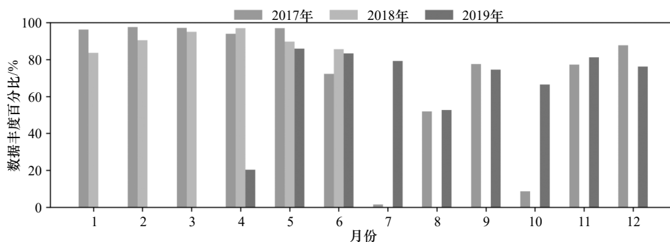
图 2 2017–2019年各月份数据丰度百分比
