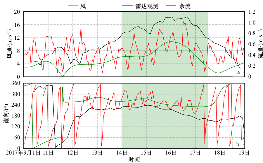
图 10 2017 年 9 月风速、余流流速、实际流速对比(a)和风向、余流流向、实际流向对比(b)
