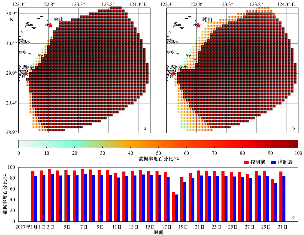
图3 质量控制前后数据丰度对比
