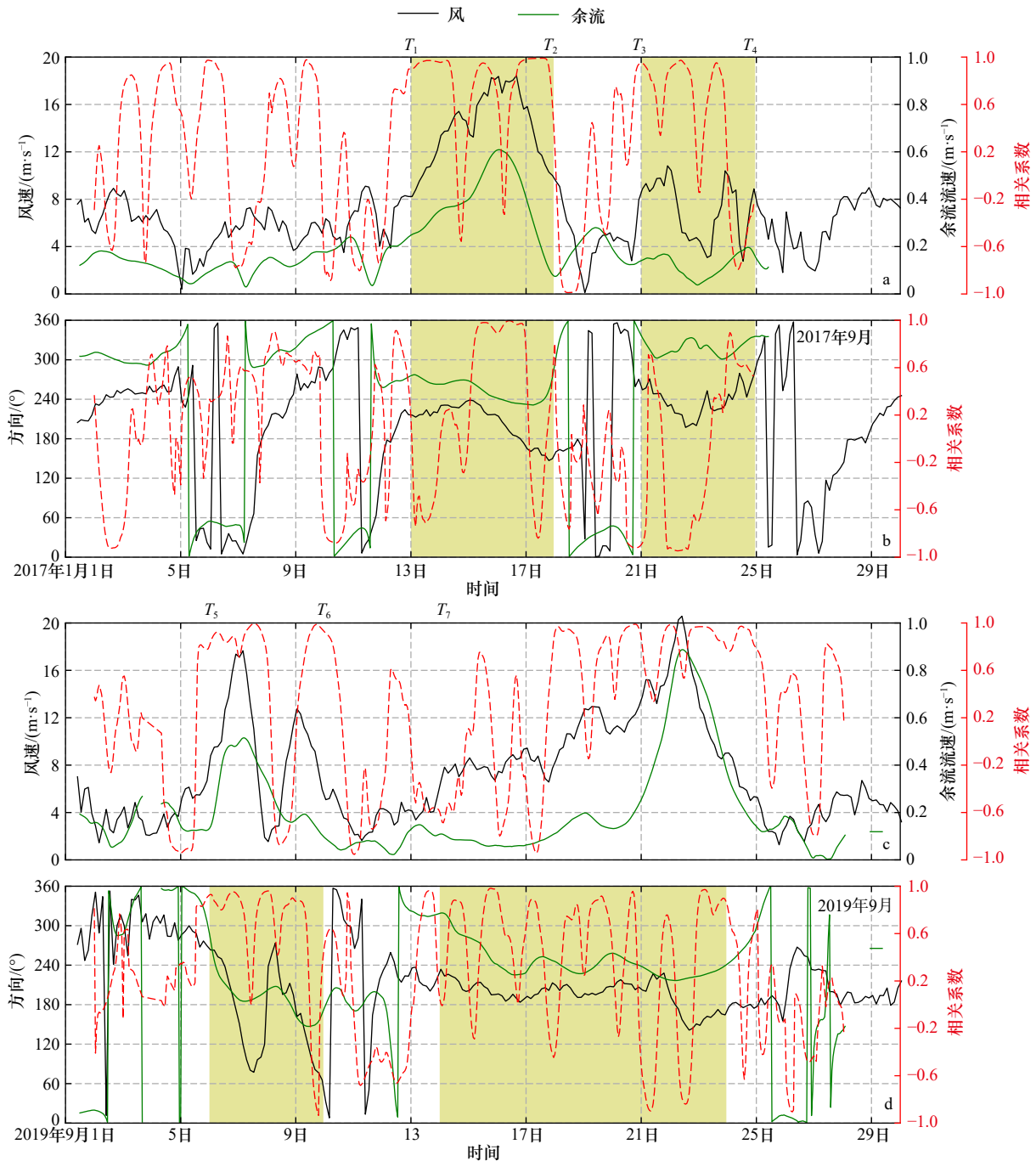
图 8 2017 年与 2019 年秋季余流与风的时间序列对比和相关系数
