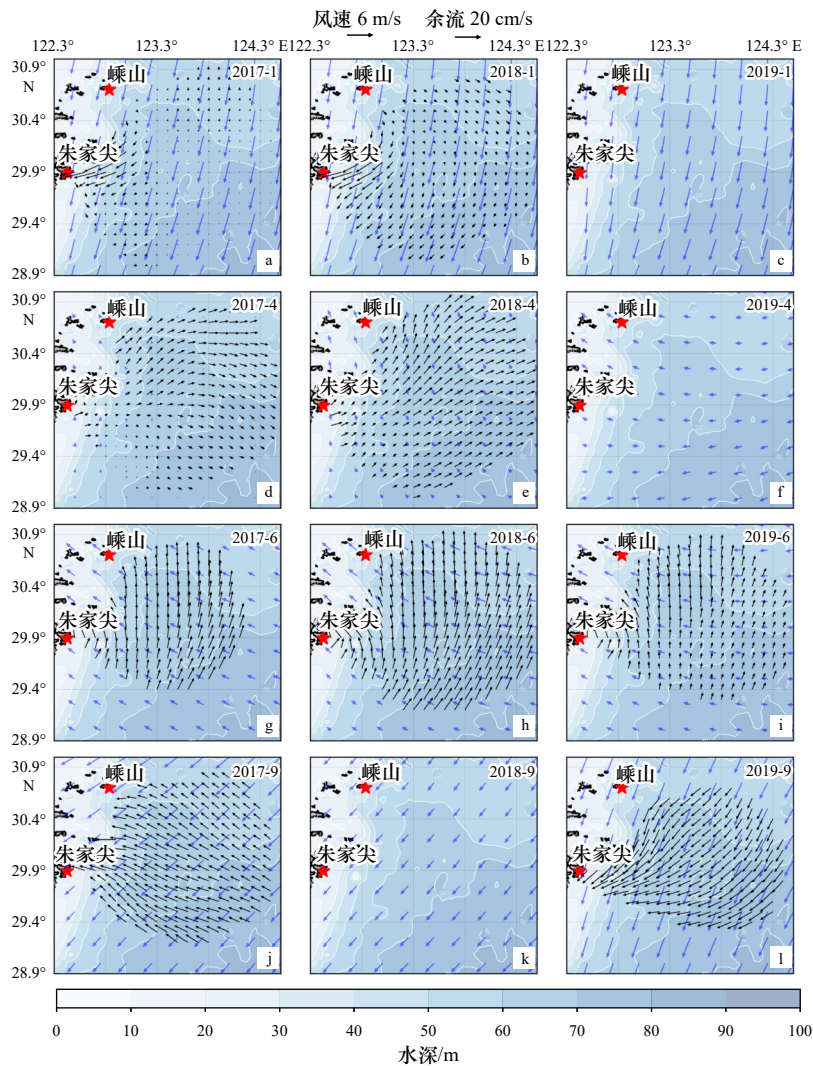
图 7 各月平均余流与风场
