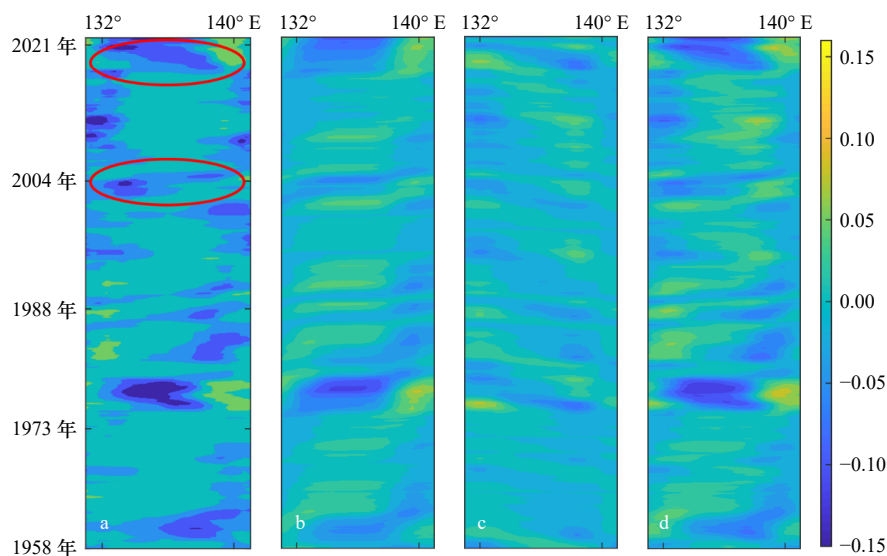
图 4 日本以南黑潮路径的霍夫默勒图(无量纲)
