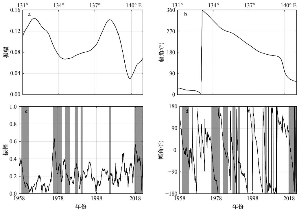
图 3 第二主模态空间分布与时间序列的振幅(无量纲)和幅角
