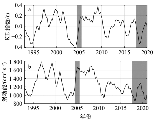
图 9 KE 指数(a)和 KE 区域(b)的涡动能时间序列 Fig. 9 KE index (a) and Eddy kinetic energy time series in the KE region (b)
