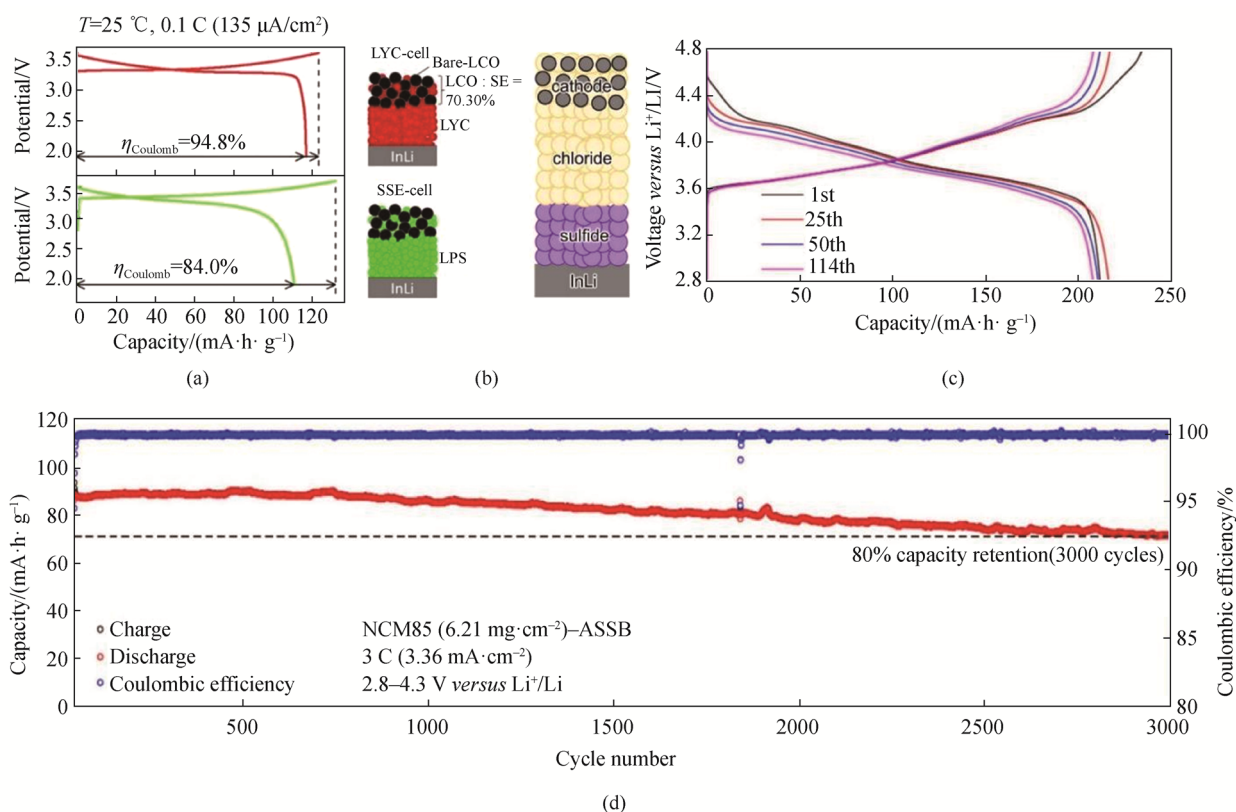
图 1 氯化物基固体电解质的高电压正极相容性 (a) \text{LiCoO}_2 正极分别匹配 \text{Li}_3\text{YCl}_6 和 \text{Li}_2\text{S-P}_2\text{S}_5 的首圈库伦效率对比 [10] 。(b) 基于氯化物基固体电解质的全固态锂离子电池典型内部结构, 其中, 包含了负极端的硫化物固体电解质缓冲层。(c) 匹配 \text{Li}_2\text{In}_{1/3}\text{Sc}_{1/3}\text{Cl}_4 的 NCM85 高镍正极以 4.8 V 为充电截止电位的电压曲线 [23] 。(d) 以 3 C 电流密度循环时匹配 \text{Li}_2\text{In}_{1/3}\text{Sc}_{1/3}\text{Cl}_4 的 NCM85 锂离子电池的超长循环寿命 [23]
