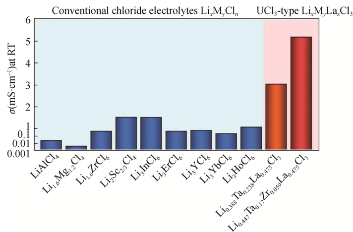
图 4 近年来报道的晶态氯化物基固体电解质室温离子电导率比较 [10–13,16,20,30,33–35]
