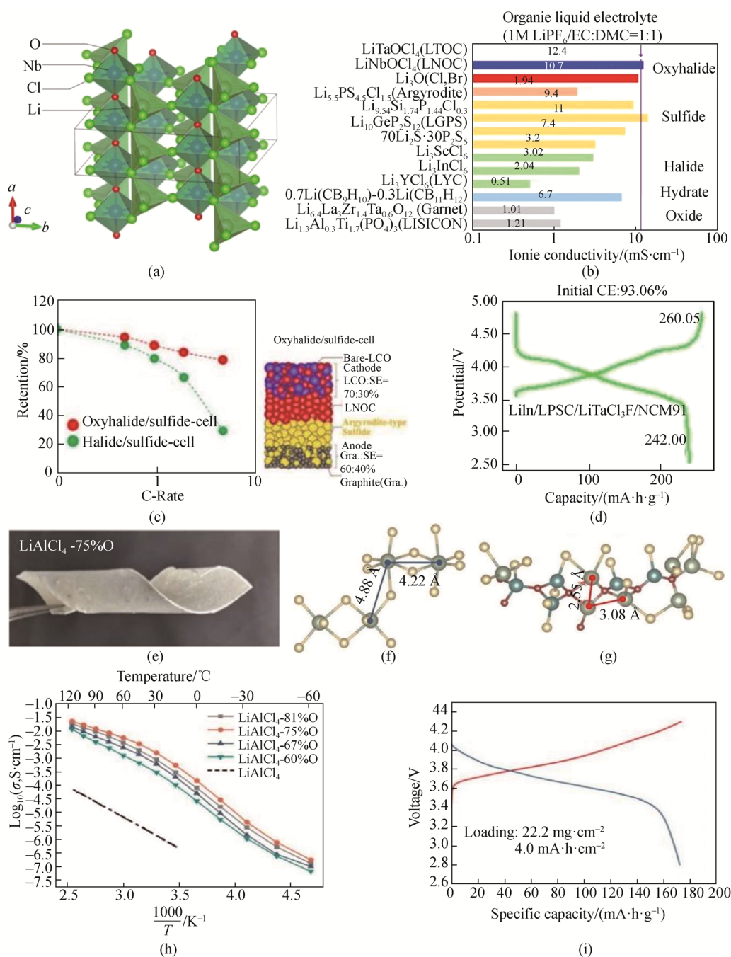
图6 阴离子取代策略提升氯化物基固体电解质性能(a) \text{LiNbOCl}_4 的晶体结构 [41] 。(b) \text{LiNbOCl}_4 (蓝色条)和一些报道过的锂离子固体电解质的室温离子电导率对比 [41] 。(c) \text{LiNbOCl}_4 /硫化物全电池和 \text{Li}_3\text{YCl}_6 /硫化物全电池的不同充放电倍率相对于0.1 C的相对放电容量对比 [41] ,同时给出了电池的內部结构示意图。(d)以LiIn合金为负极, \text{Li}_{5.4}\text{PS}_{4.4}\text{Cl}_{1.6} 为夹层, NCM91为正极, \text{LiTaCl}_3\text{F} 为电解质的全固态电池的首圈充放电曲线 [24] 。(e)通过卷曲工艺得到的 \text{LiAlCl}_{2.5}\text{O}_{0.75} 弯曲膜 [42] 。(f-g) \text{LiAlCl}_4 (f)和 \text{LiAlCl}_{2.5}\text{O}_{0.75} (g)中具有最短锂离子传导距离的结构碎片 [42] 。(h) \text{LiAlCl}_{2.5}\text{O}_{0.75} 和 \text{LiAlCl}_4 锂离子电导率随温度变化的Arrhenius曲线 [42] 。(i)采用厚正极和 \text{LiAlCl}_{2.5}\text{O}_{0.75} 固体电解质的 NCM622 电池的第3圈充放电电压曲线 [42]
