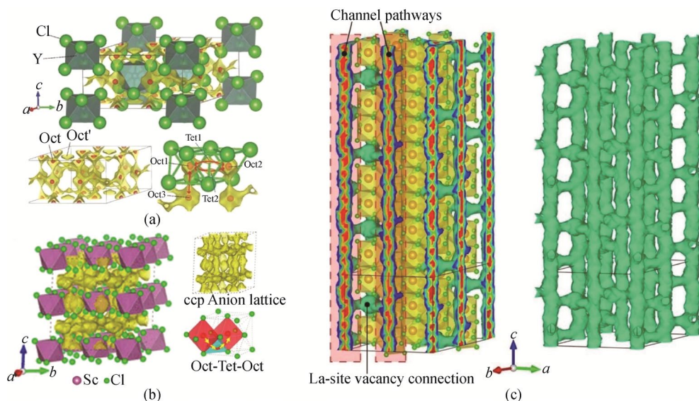
图 5 锂离子在一些典型氯化物基固体电解质中的迁移路径 (a)键价位能(BVSE)计算方法得出的 \text{Li}_3\text{YCl}_6 晶格中的锂离子势能图 [10] 。(b)通过从头算分子动力学(AIMD)模拟得到的 \text{Li}_3\text{ScCl}_6 晶格中的锂离子概率密度等值面 [14] 。(c)AIMD 模拟得到的含镧空位的 \text{LaCl}_3 晶格中的锂离子概率密度等值面 [27]
