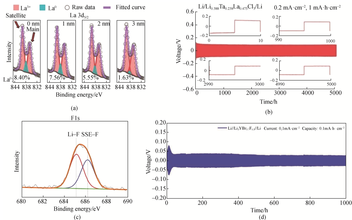
图 3 与锂金属负极界面更稳定的氯化物基固体电解质(a)50 h 循环后, 不同深度下 \text{Li}_{0.388}\text{Ta}_{0.238}\text{La}_{0.475}\text{Cl}_3 固体电解质界面 \text{La } 3d_{5/2} 的 XPS 谱 [29] 。(b)30 °C 时 \text{Li}/\text{Li}_{0.388}\text{Ta}_{0.238}\text{La}_{0.475}\text{Cl}_3/\text{Li} 对称电池在电流密度 0.2 \text{ mA}/\text{cm}^2 和面容量 1 \text{ mAh}/\text{cm}^2 下循环的电压曲线。(c) \text{Li}/\text{Li}_3\text{YBr}_{5.7}\text{F}_{0.3}/\text{Li} 界面 \text{F } 1s 的 XPS 谱 [31] 。(d) \text{Li}/\text{Li}_3\text{YBr}_{5.7}\text{F}_{0.3}/\text{Li} 对称电池在电流密度 0.1 \text{ mA}/\text{cm}^2 和面容量 0.1 \text{ mAh}/\text{cm}^2 下循环时的电压曲线 [31]
