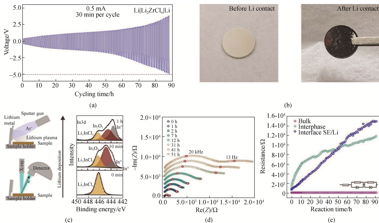
图2 氯化物基固体电解质对金属锂负极的界面不稳定性 (a)0.5 mA 条件下 \text{Li}/\text{Li}_2\text{ZrCl}_6/\text{Li} 对称电池的恒流循环曲线(每个沉积/脱出循环 30 min) [29] 。(b) \text{Li}_2\text{ZrCl}_6 片在接触锂金属 240 h 前后的照片 [29] 。(c) \text{Li}_3\text{InCl}_6 与金属锂接触的过程中, \text{In}3d 的 XPS 谱 [28] 。(d–e) \text{Li}|\text{Li}_3\text{InCl}_6|\text{Li} 对称电池的阻抗响应随时间变化曲线(d), 以及不同反应时间的电阻随时间变化曲线(e) [28]
