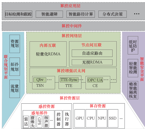
图1 算控网络架构
