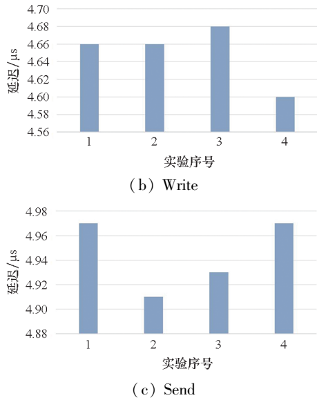
图3 不同传输模式的延迟测试结果
