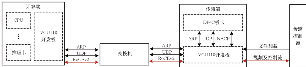
图 2 轻量化 RDMA 验证平台 Fig. 2 Lightweight RDMA verification platform
