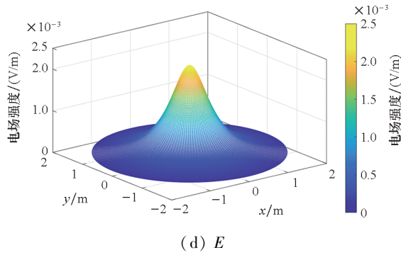
图 6 平行于圆盘平面上的电场分布
