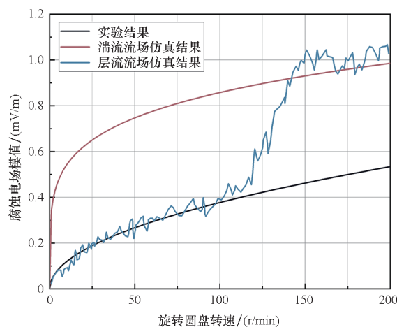
图8 仿真与实验结果对比
