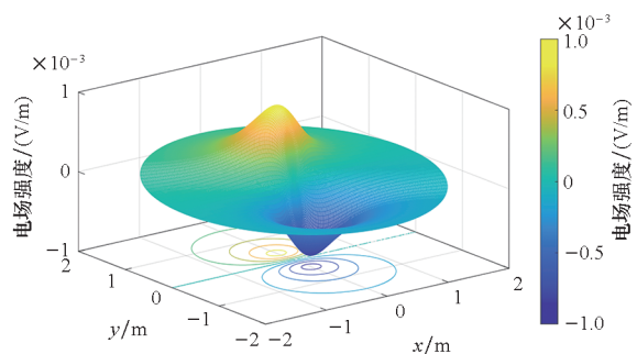
(b) E_y
