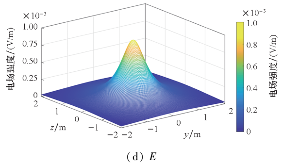
图 7 垂直于圆盘平面上的电场分布
