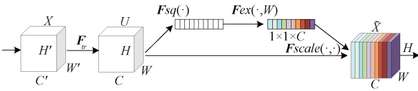
图 3 SE 注意力模块
