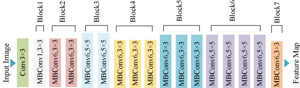
图 2 EfficientNet 模型架构
