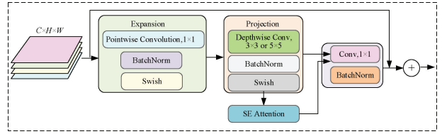
图 4 MBCConv 结构
