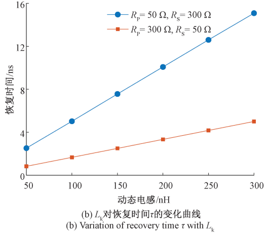
图 8 各参数对探测器恢复时间的影响
